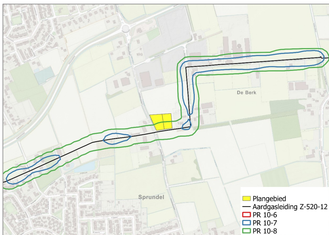
Figuur 3. Plaatsgebonden risicocontouren aardgasleiding Z-520-12 Gasunie
