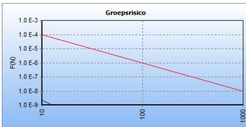
Figuur 4. Groepsrisico Z-520-12, huidig en toekomstig
