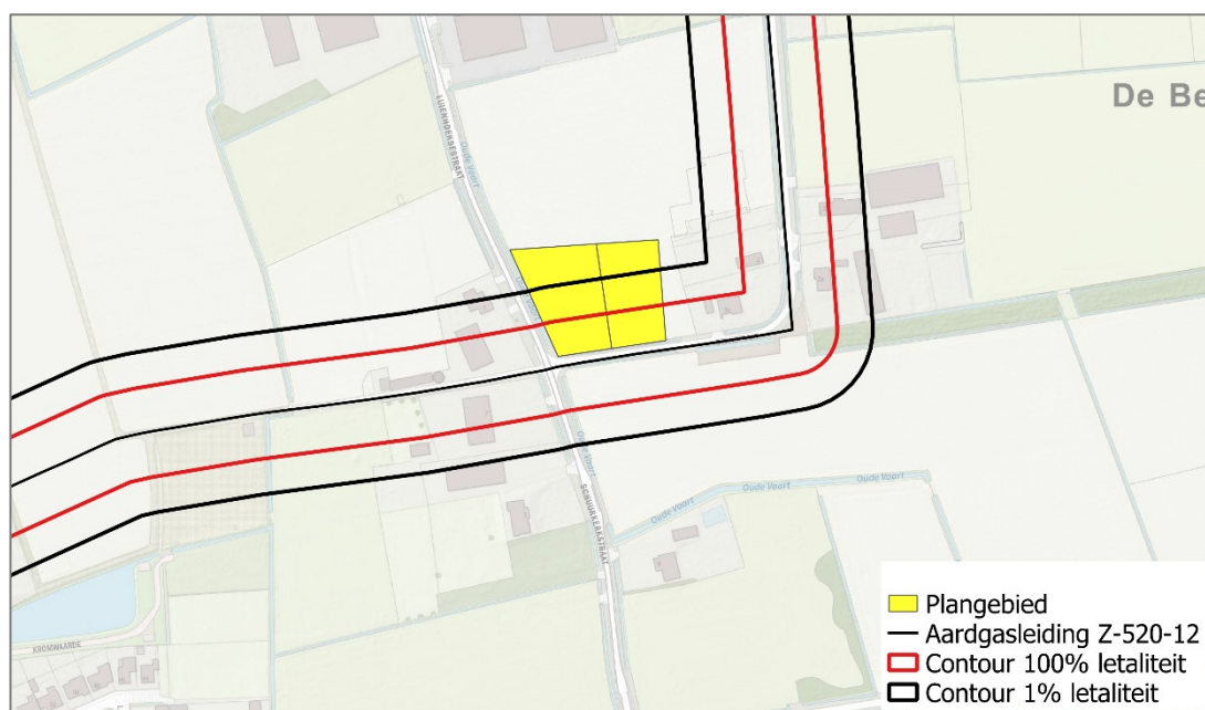
Figuur 2. Invloedsgebied en 100%-letaliteitscontour aardgasleiding Z-520-12
