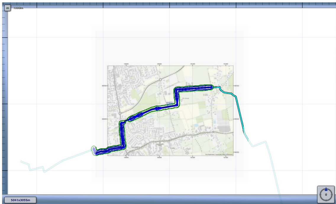
3.1 Figuur 3.2 Plaatsgebonden risico voor 5853_leiding-Z-520-12-deel-1 van N.V. Nederlandse Gasunie
