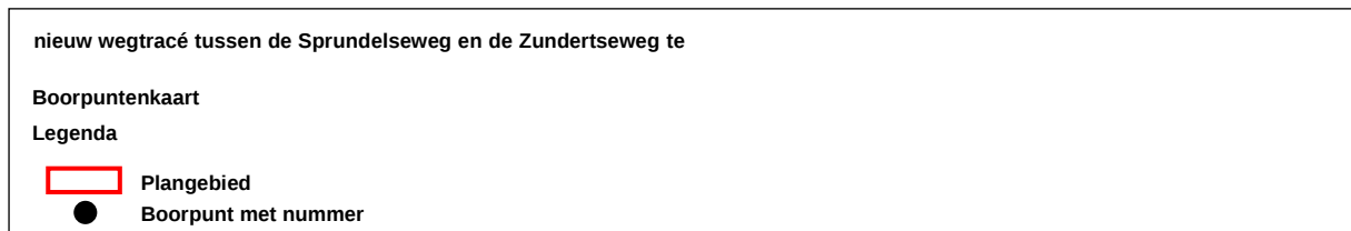
Figuur 11. Boorpuntenkaart
