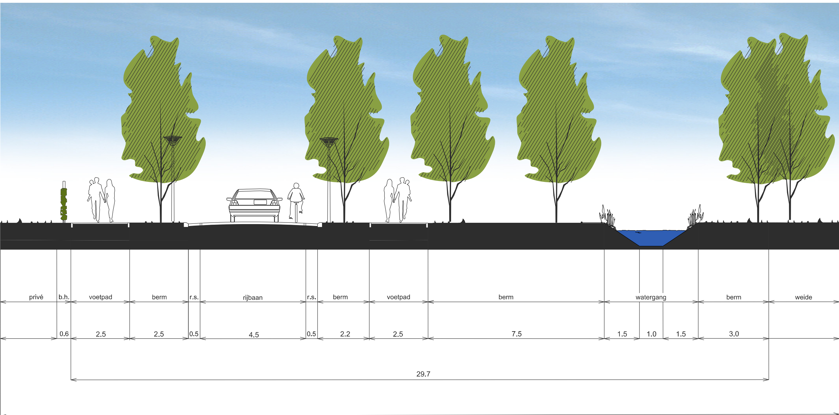
PROFIEL 14
