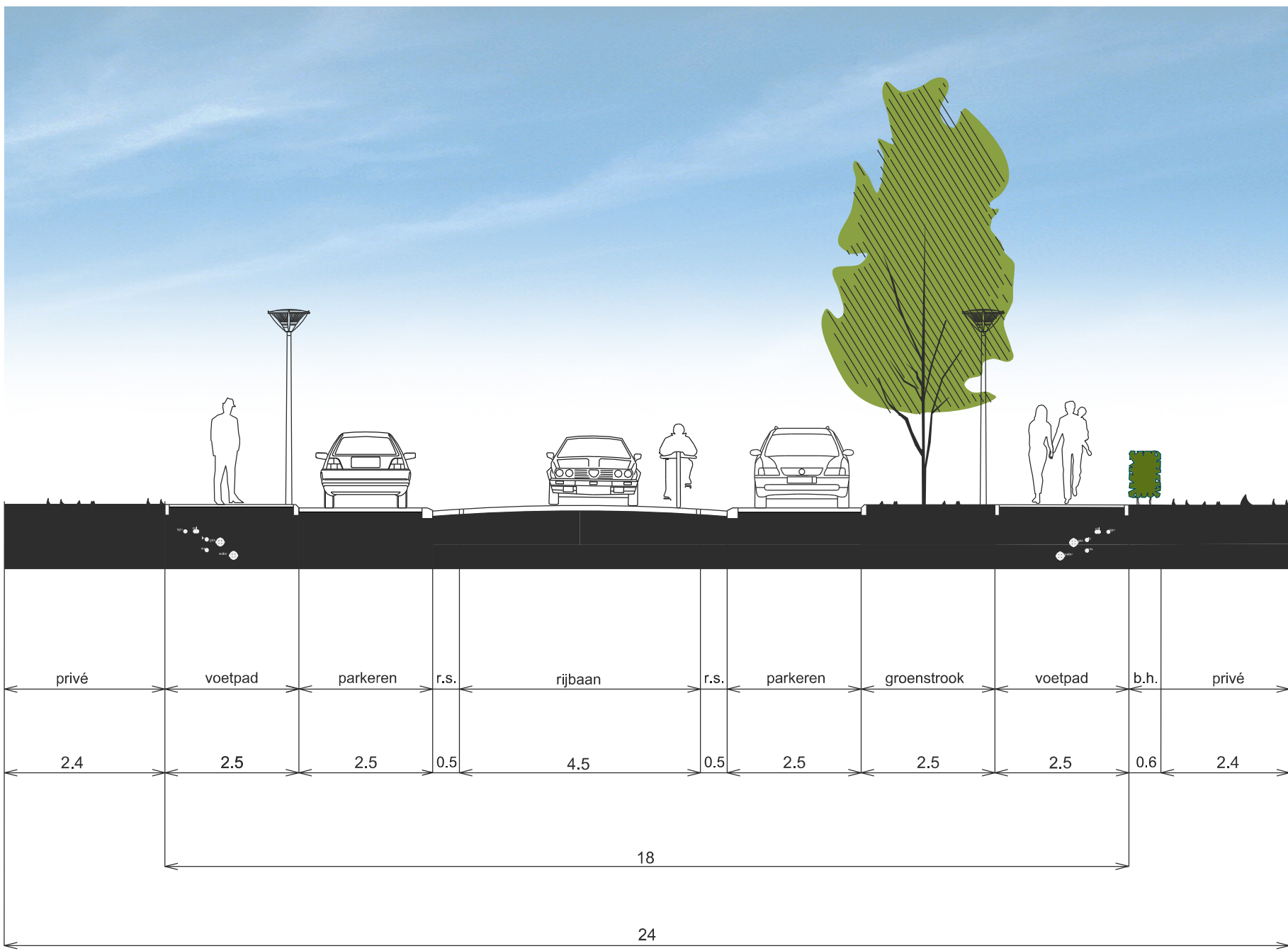
PROFIEL 5
