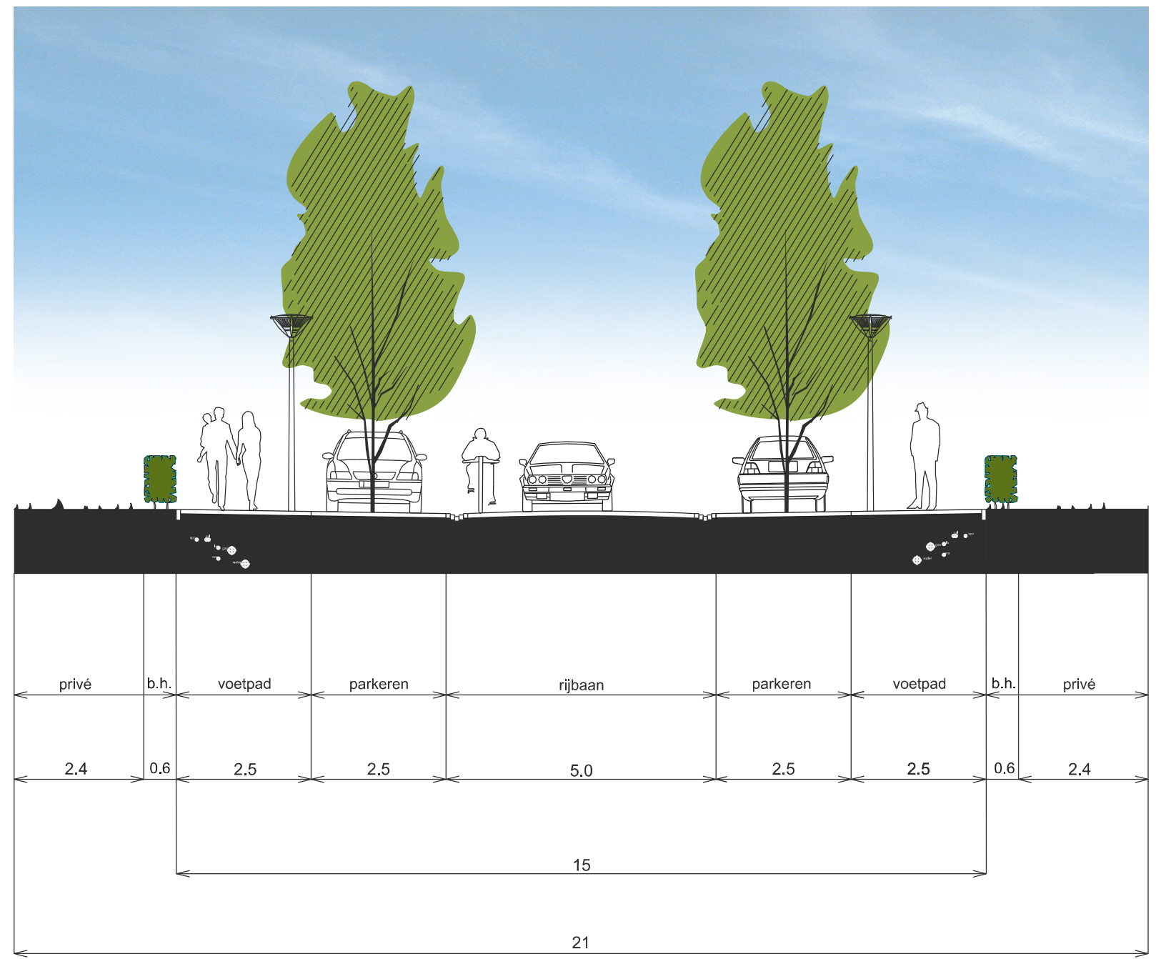
PROFIEL 9
