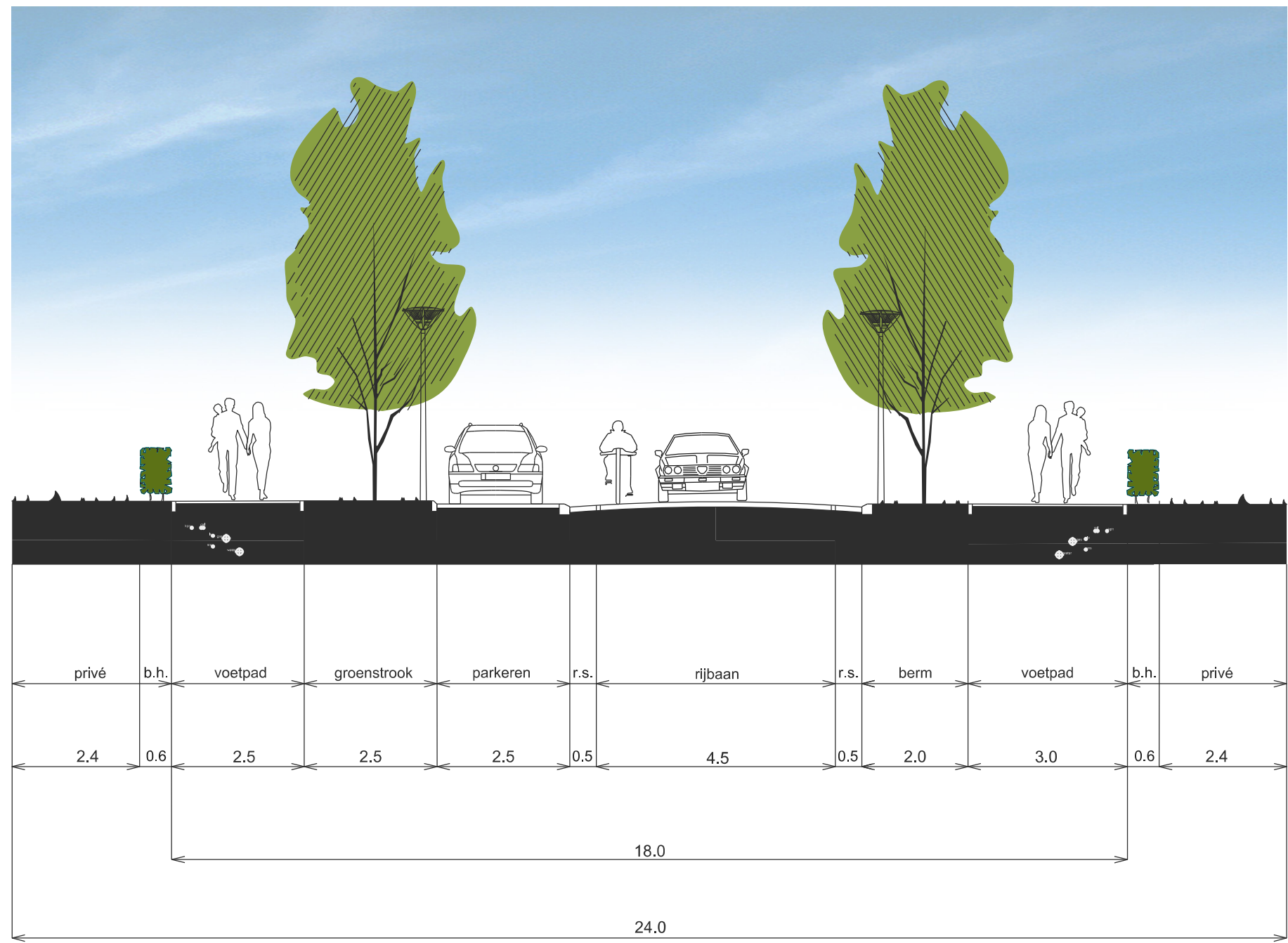
PROFIEL 4
