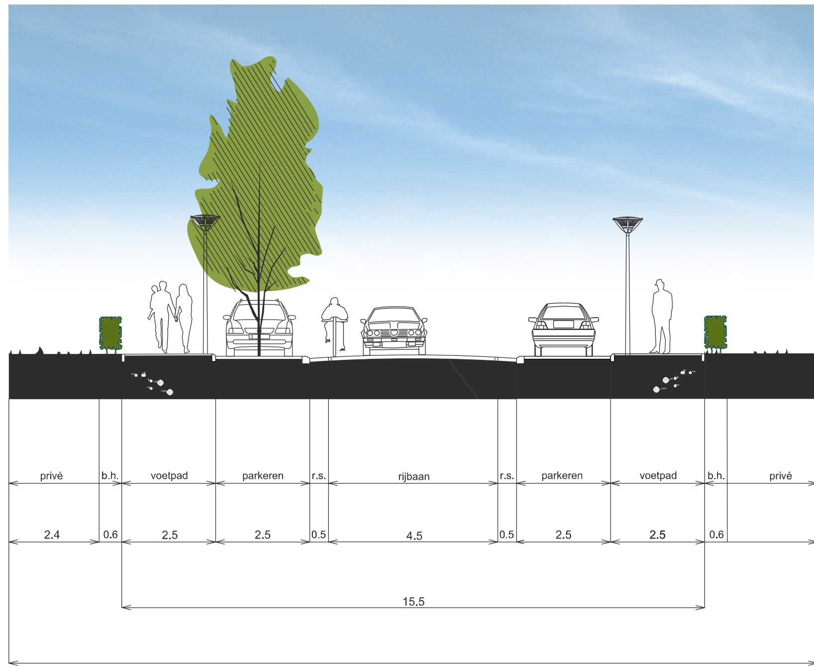
PROFIEL 6
