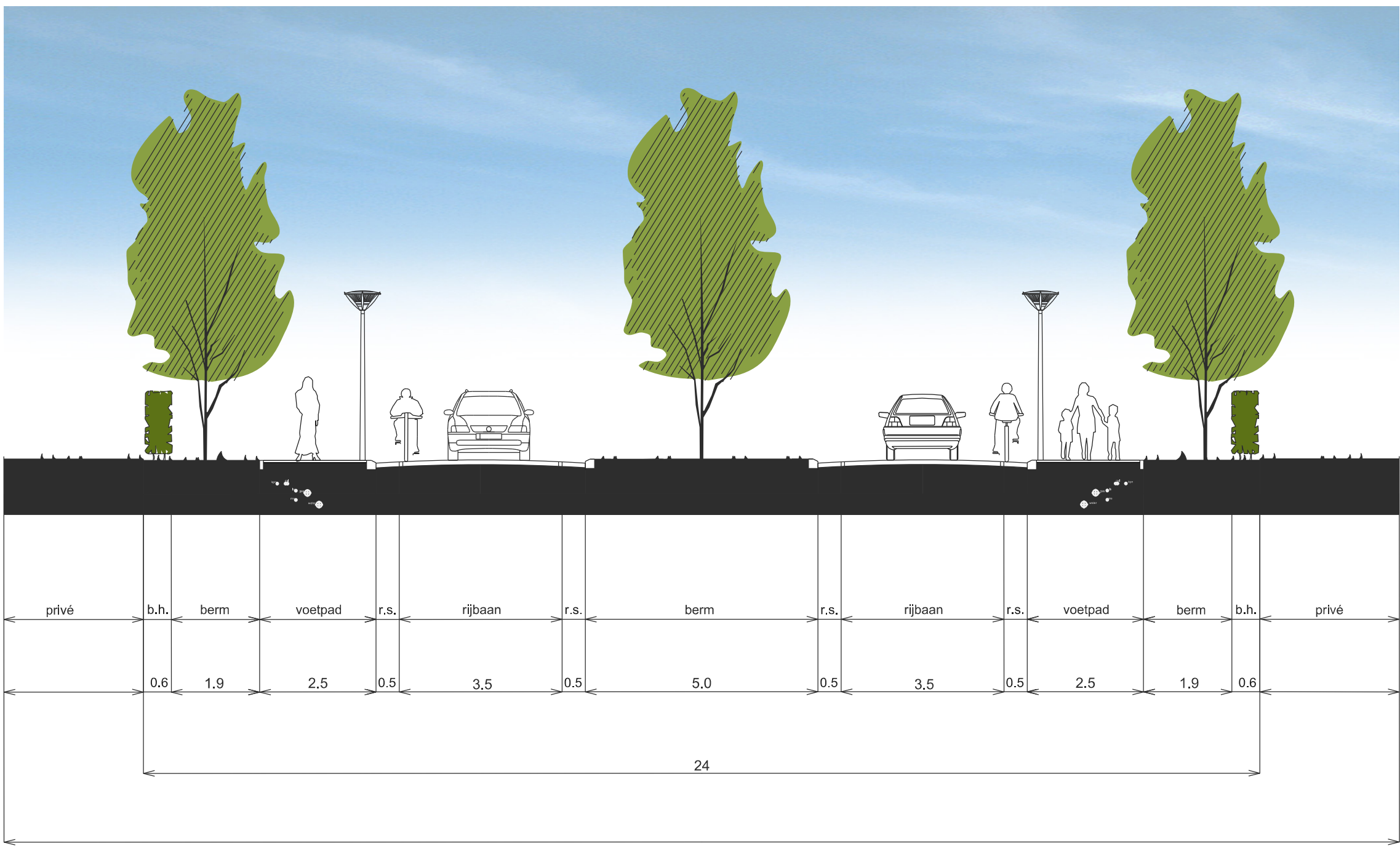
PROFIEL 1
