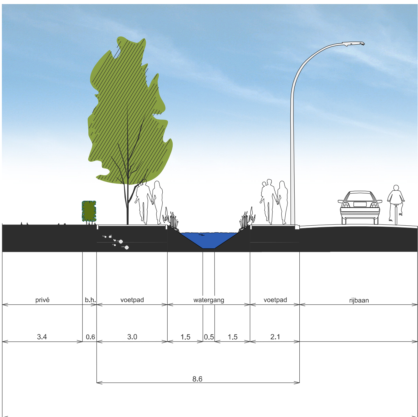
PROFIEL 23 - KERKSTRAAT
