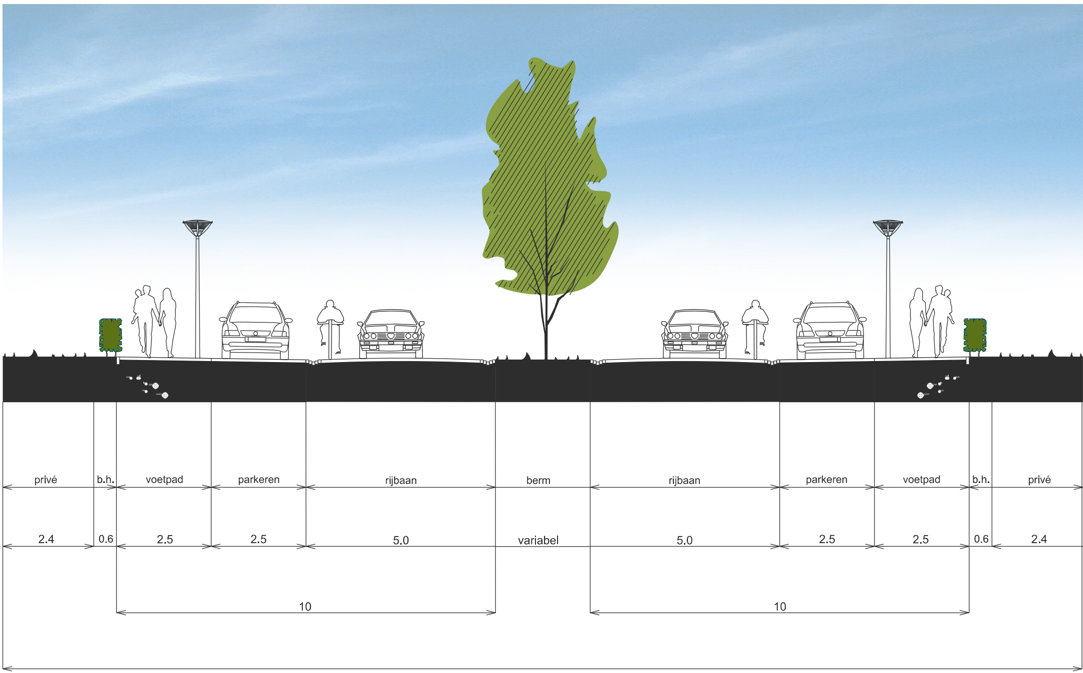
PROFIEL 10
