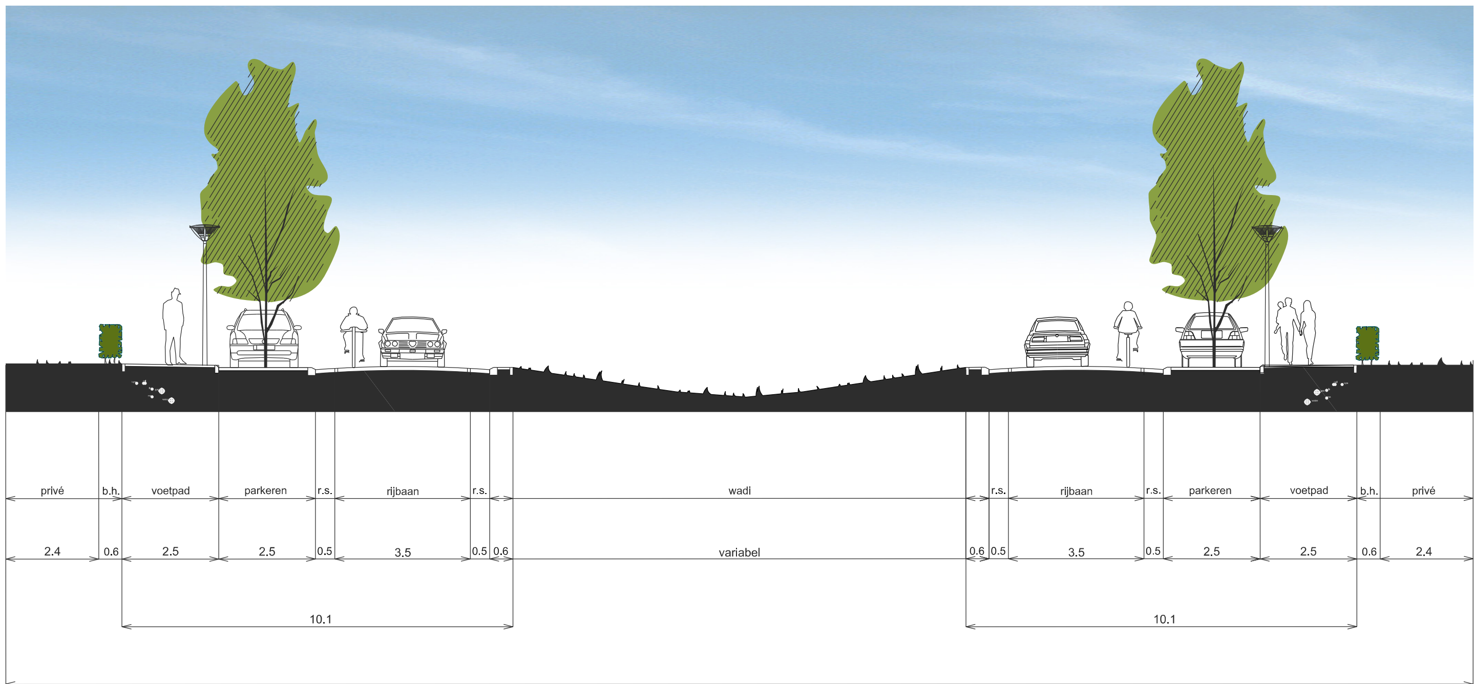
PROFIEL 18
