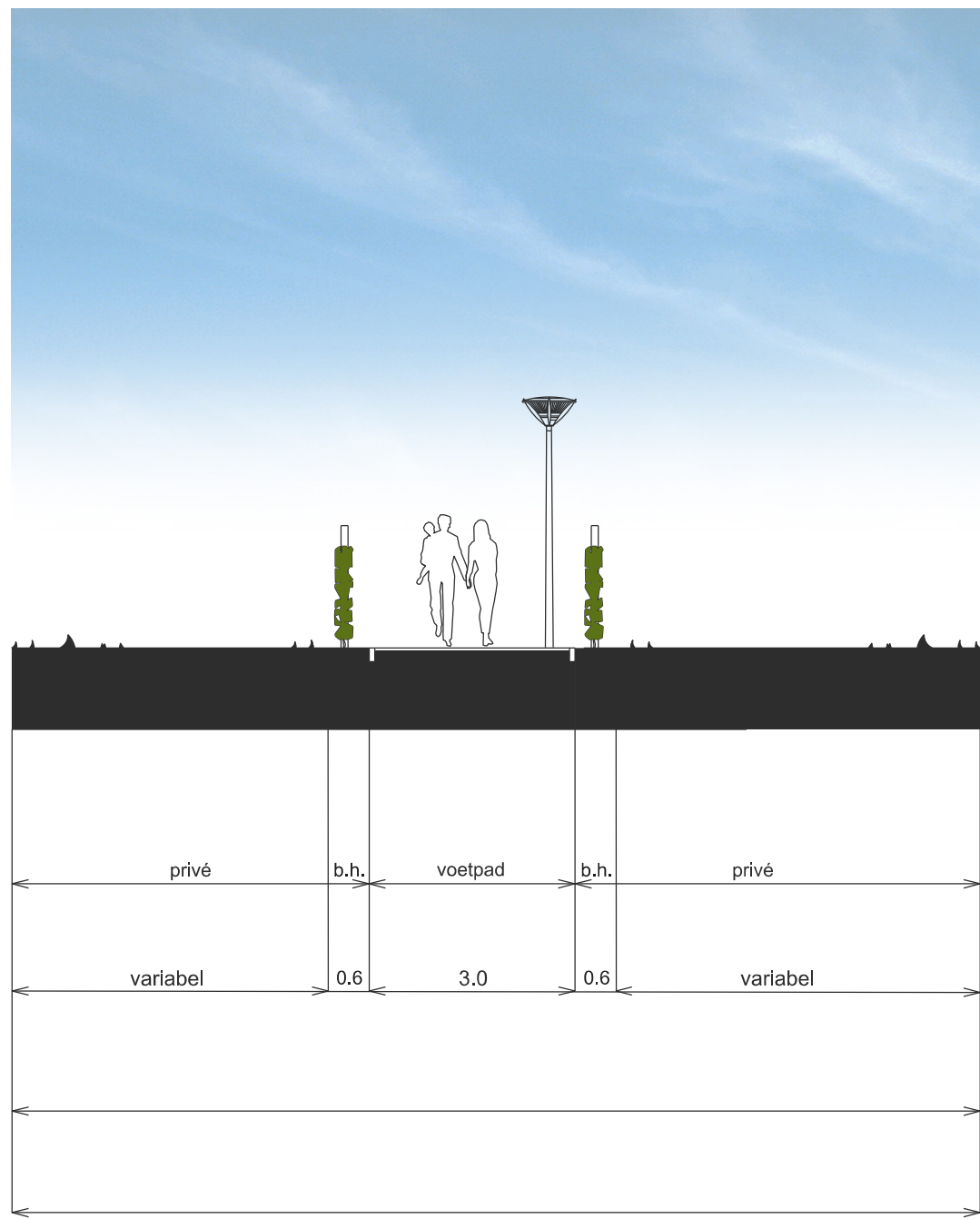
PROFIEL 3
