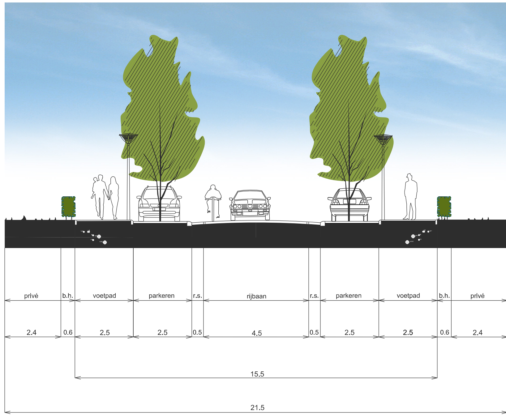
PROFIEL 11
