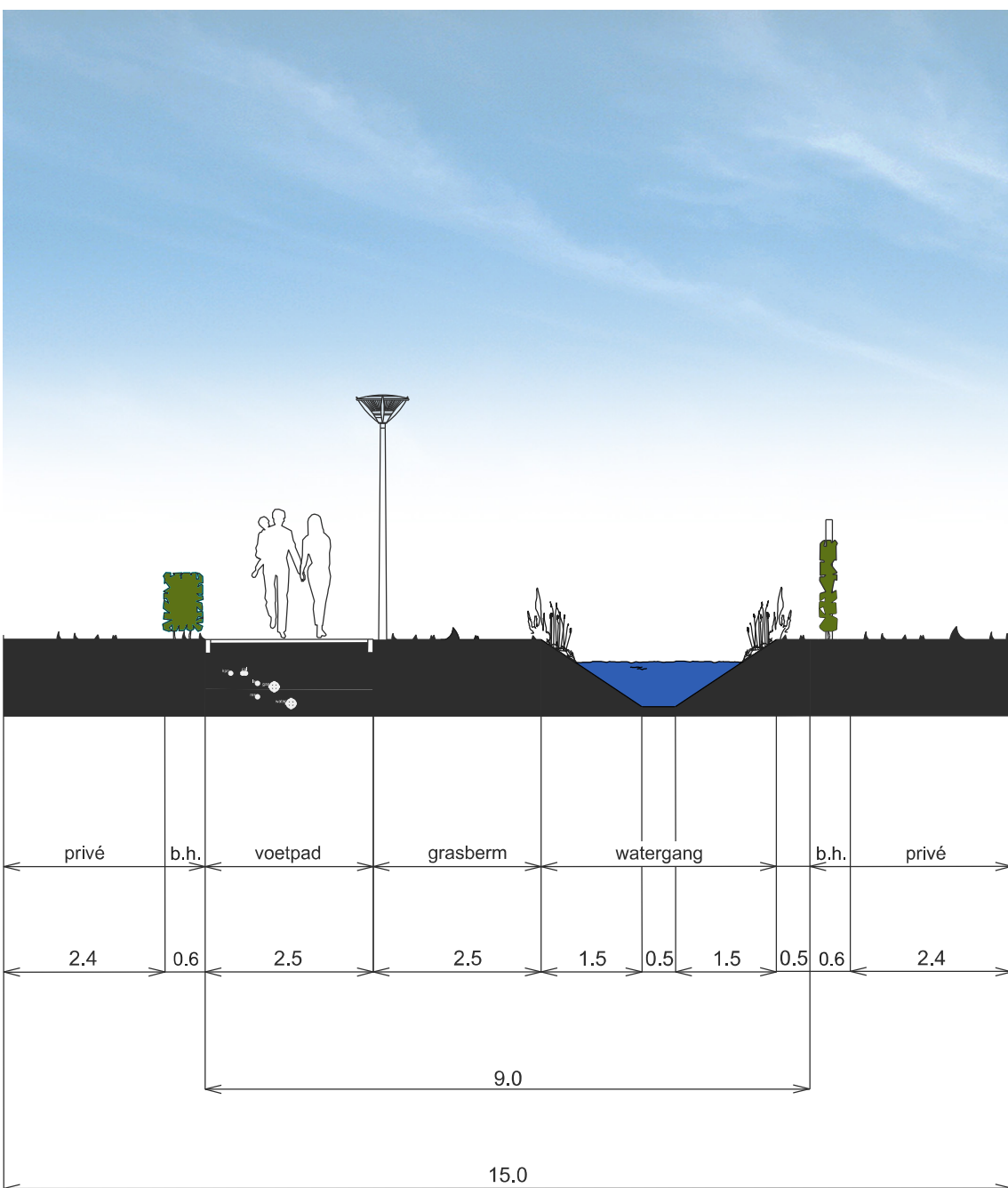
PROFIEL 17
