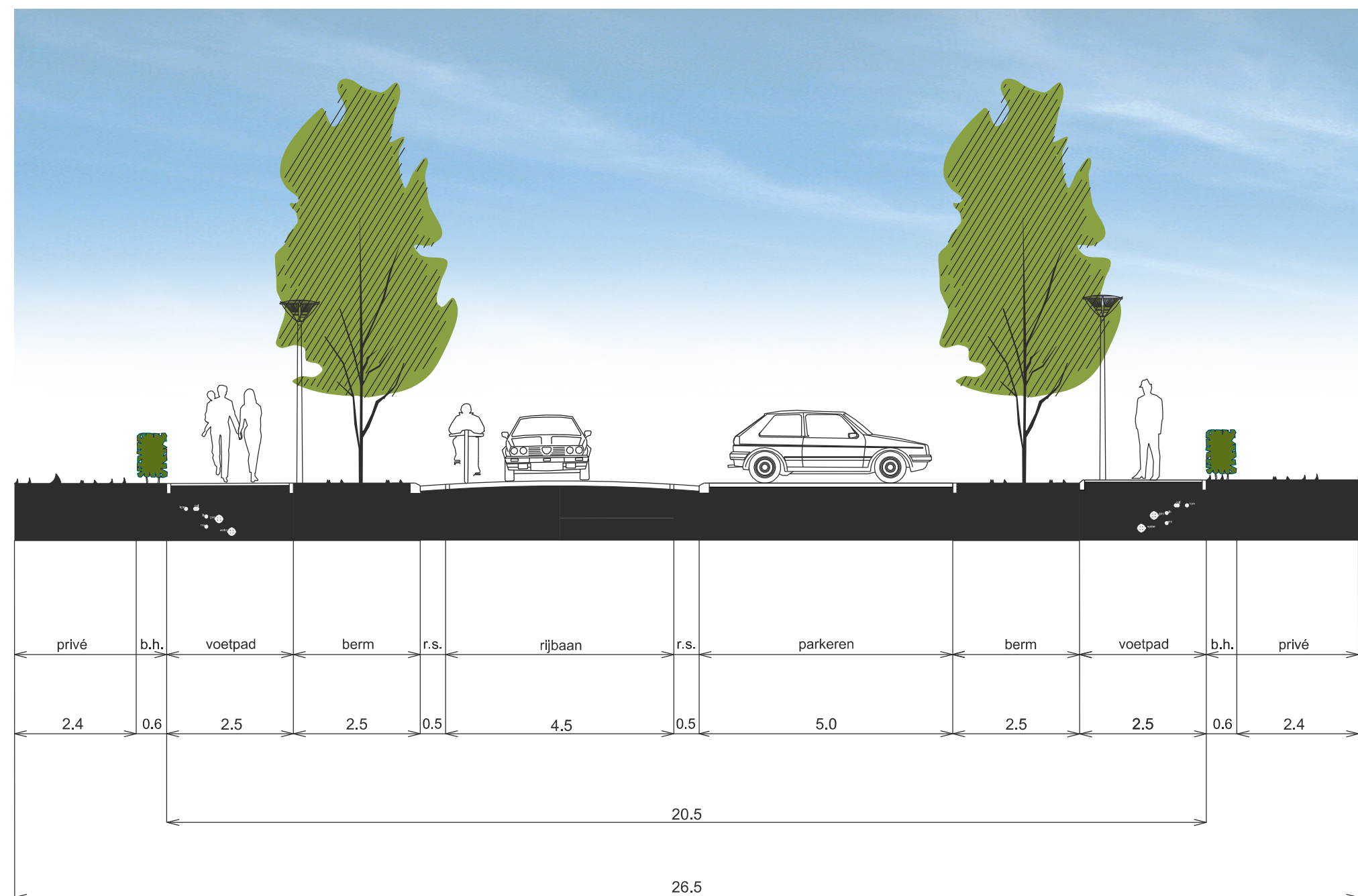
PROFIEL 22
