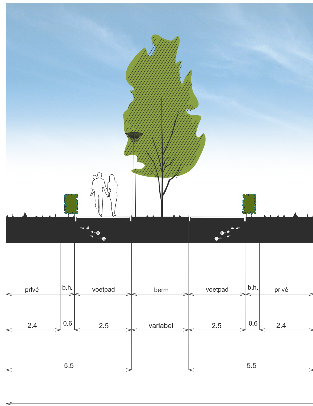
PROFIEL 8
