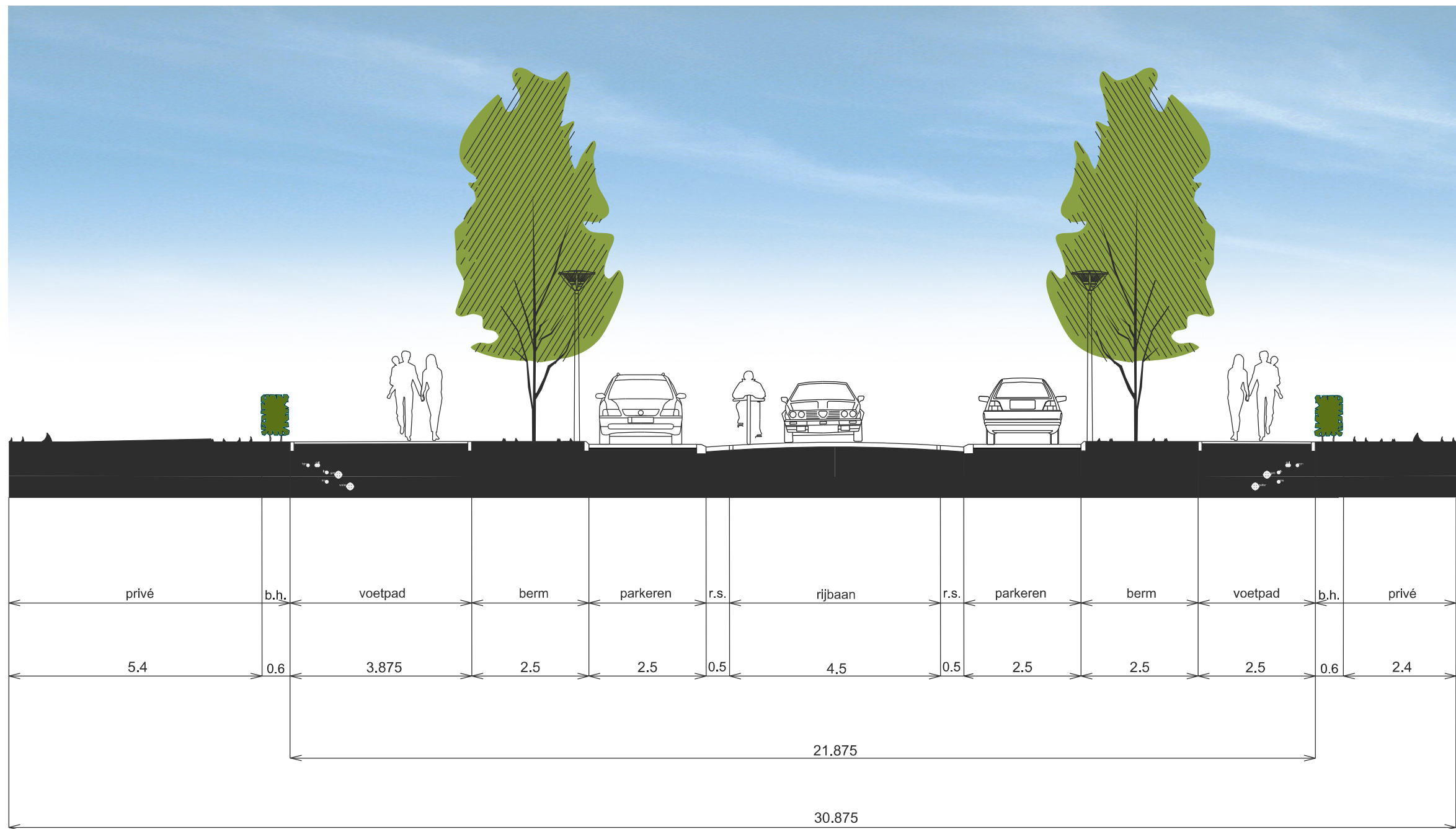
PROFIEL 16
