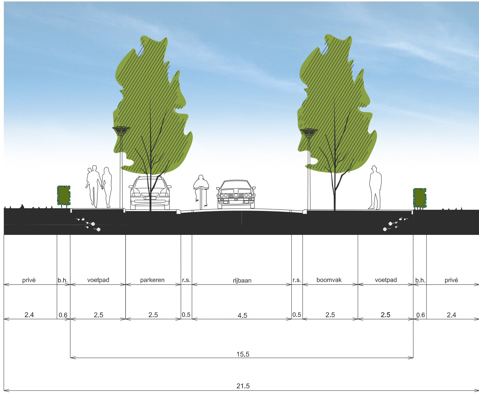
PROFIEL 13
