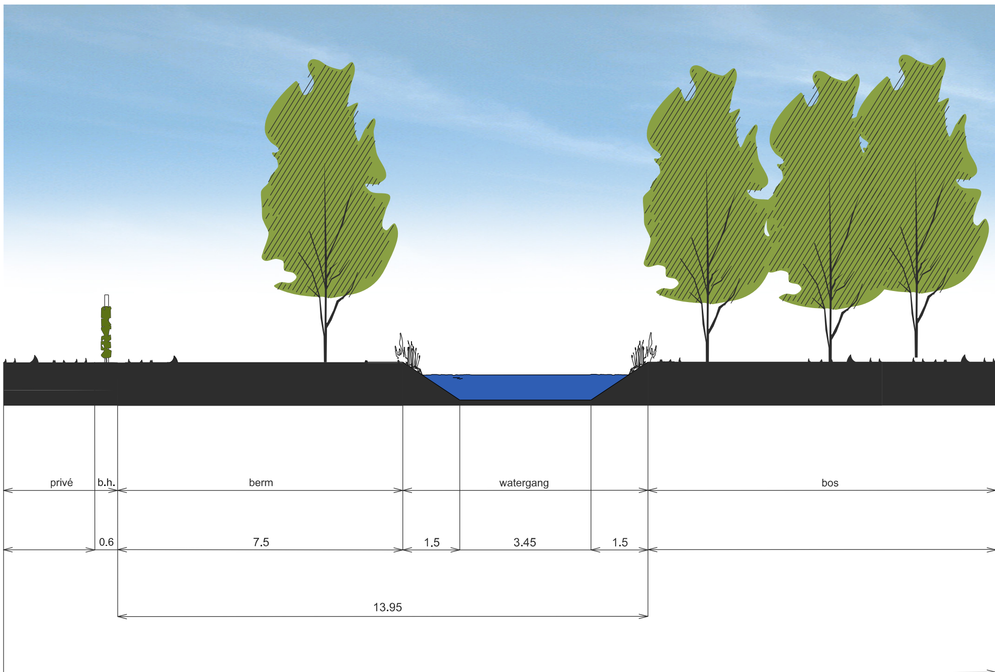
PROFIEL 15
