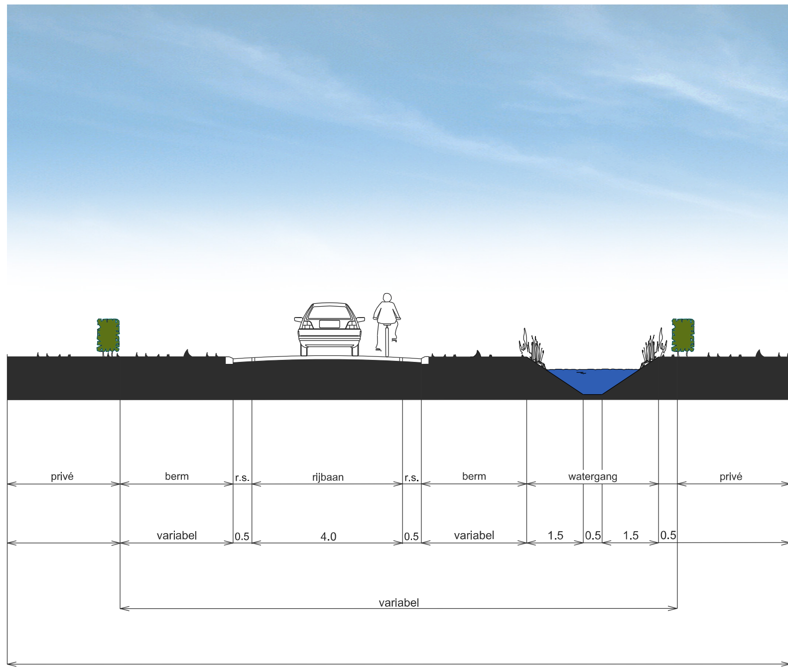
PROFIEL 7 - PIERESTRAAT
