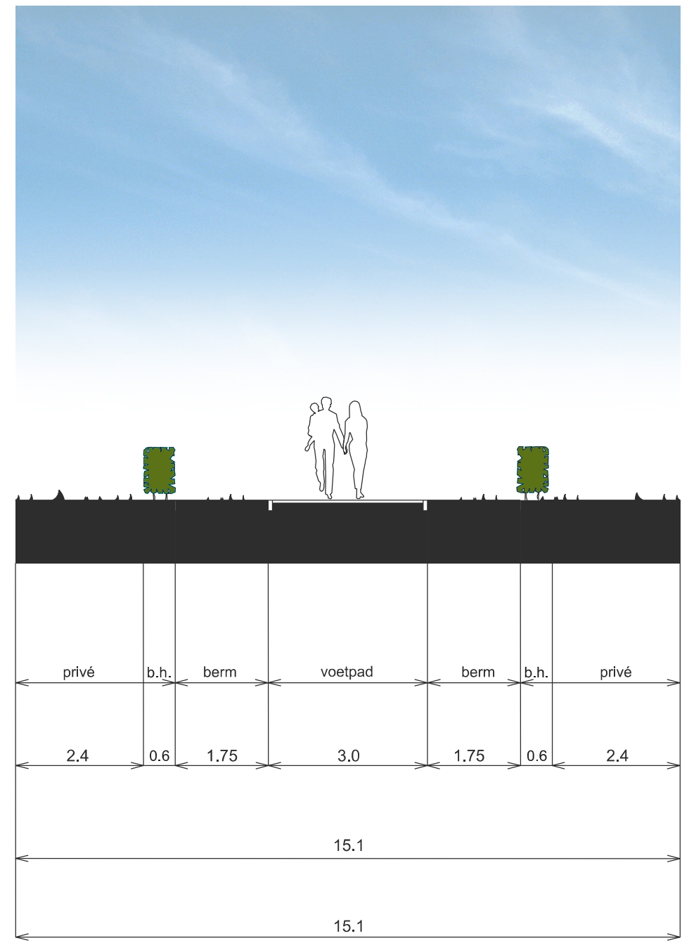
PROFIEL 12
