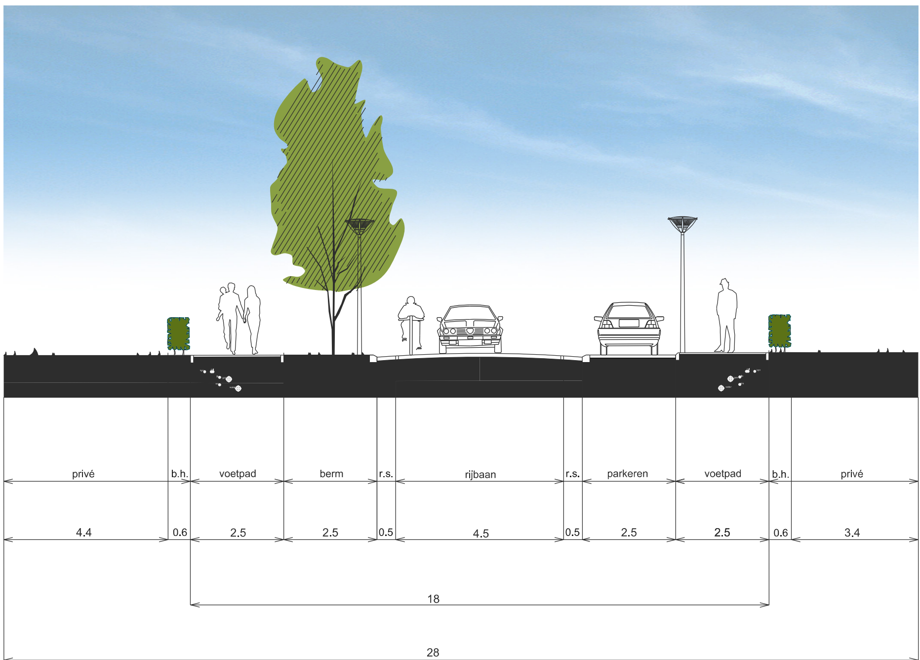
PROFIEL 20
