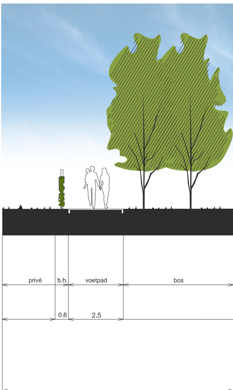
PROFIEL 24
