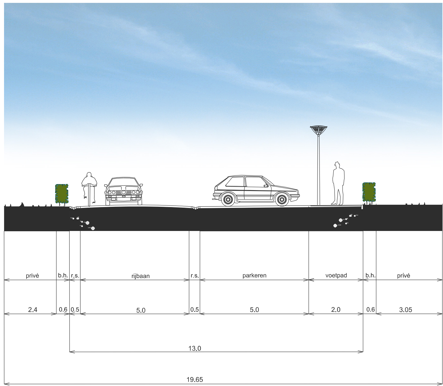
PROFIEL 2
