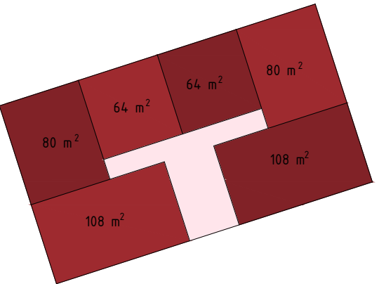
3e Bouwlaag
