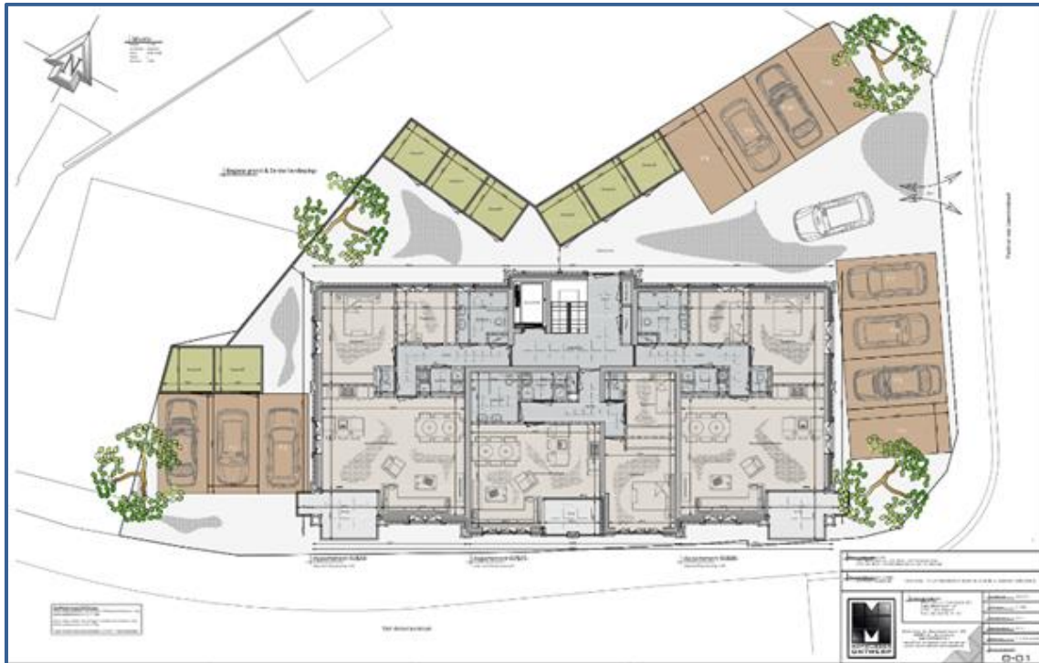
Afbeelding 2. Ontwerptekening beoogde situatie
