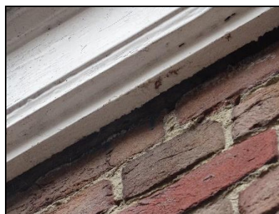
Figuur 7. Detail ruimte onder boeiboorden woonhuis,
