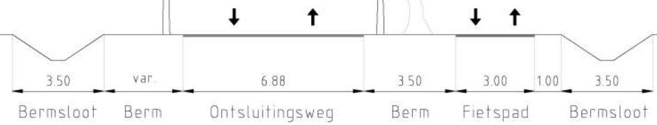
Profiel schaal: 1:200
