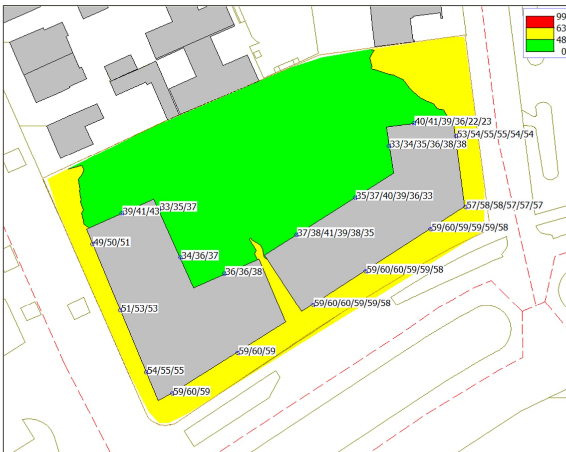
Afbeelding 8 Geluidbelasting ten gevolge van de Hertogensingel inclusief afrek artikel 110g Wvgh
