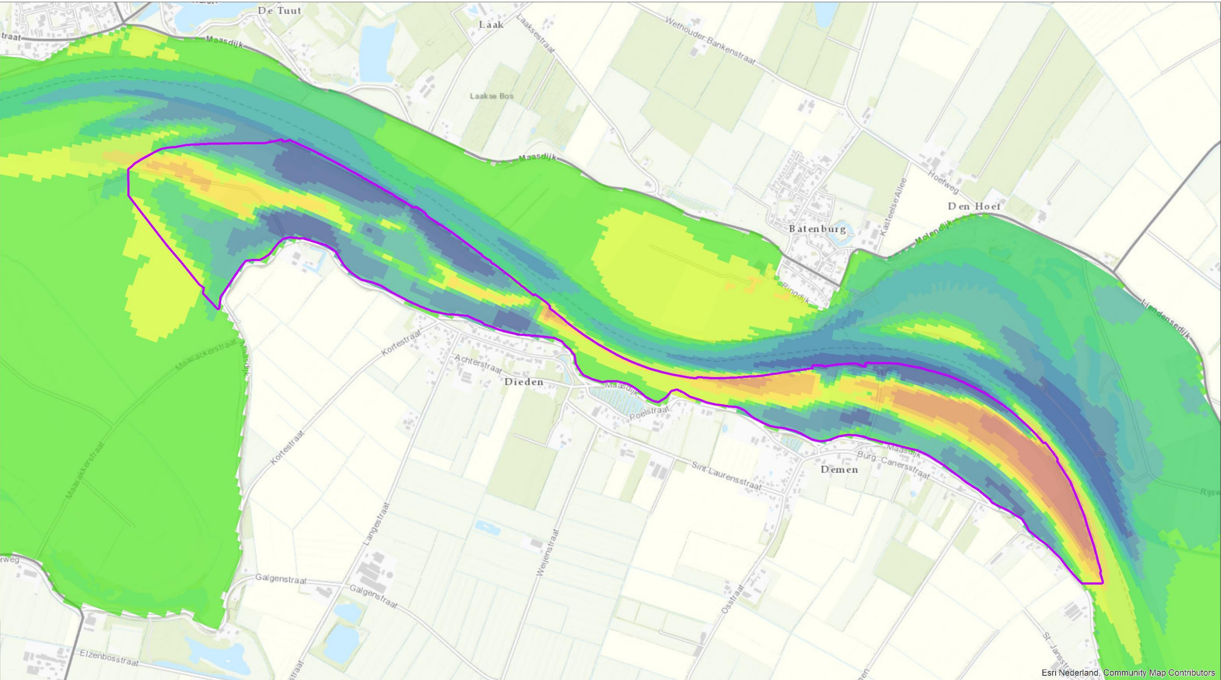
Stroomsnelheidsverschil [m/s] bij 4.000 m³/s
