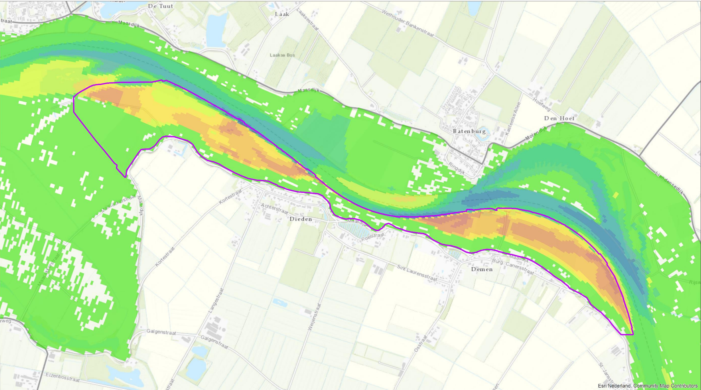
Stroomsnelheidsverschil [m/s] bij 1.500 m³/s
