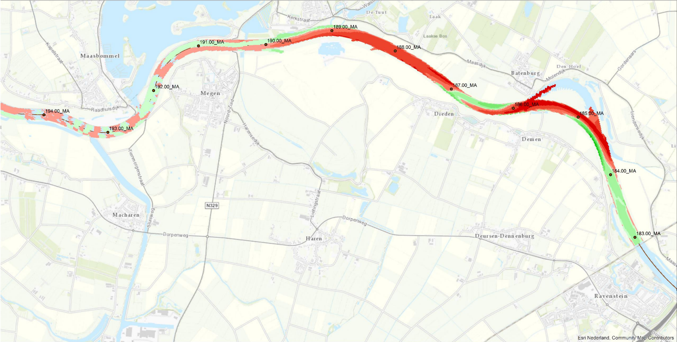
Jaargemiddeld morfologisch effect in meters
