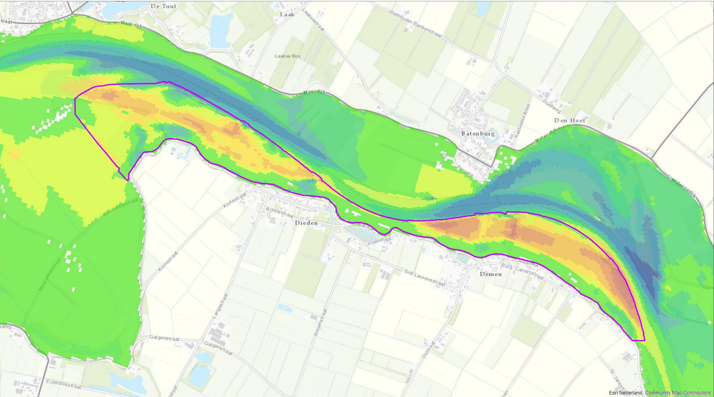
Stroomsnelheidsverschil [m/s] bij 2.000 m³/s
