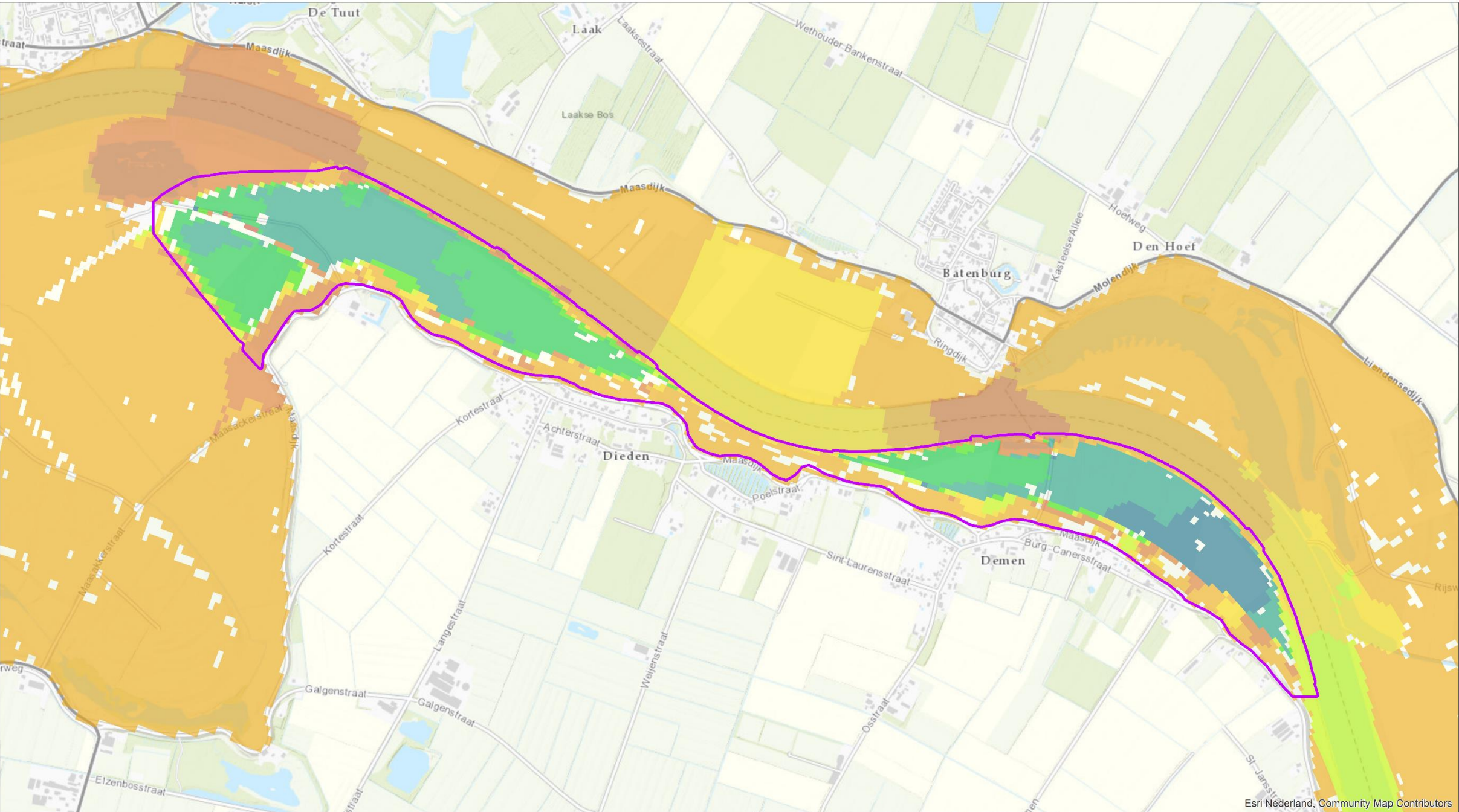
Waterstandverschillen [m] bij 1.500 m³/s
