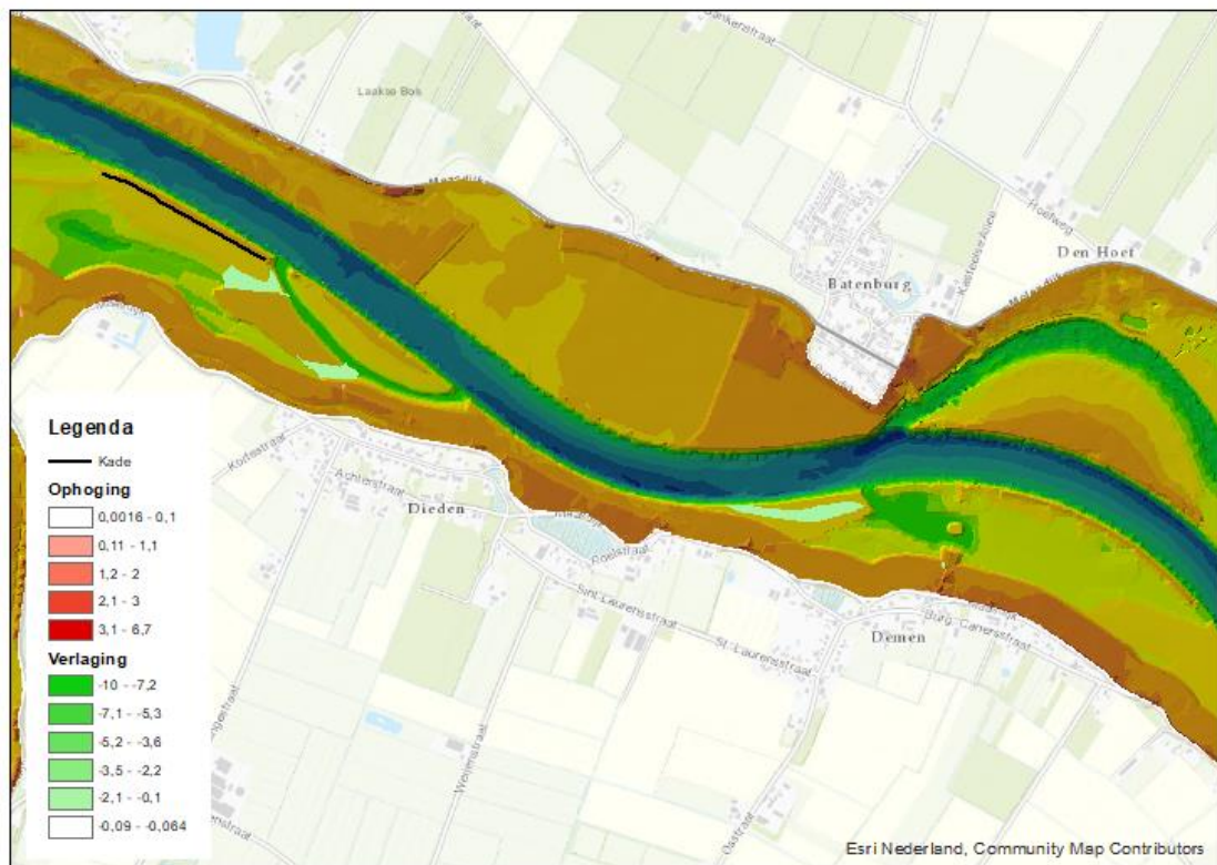
Figuur 10: Wijzigingen derde optimalisatieslag t.o.v. tweede optimalisatieslag
