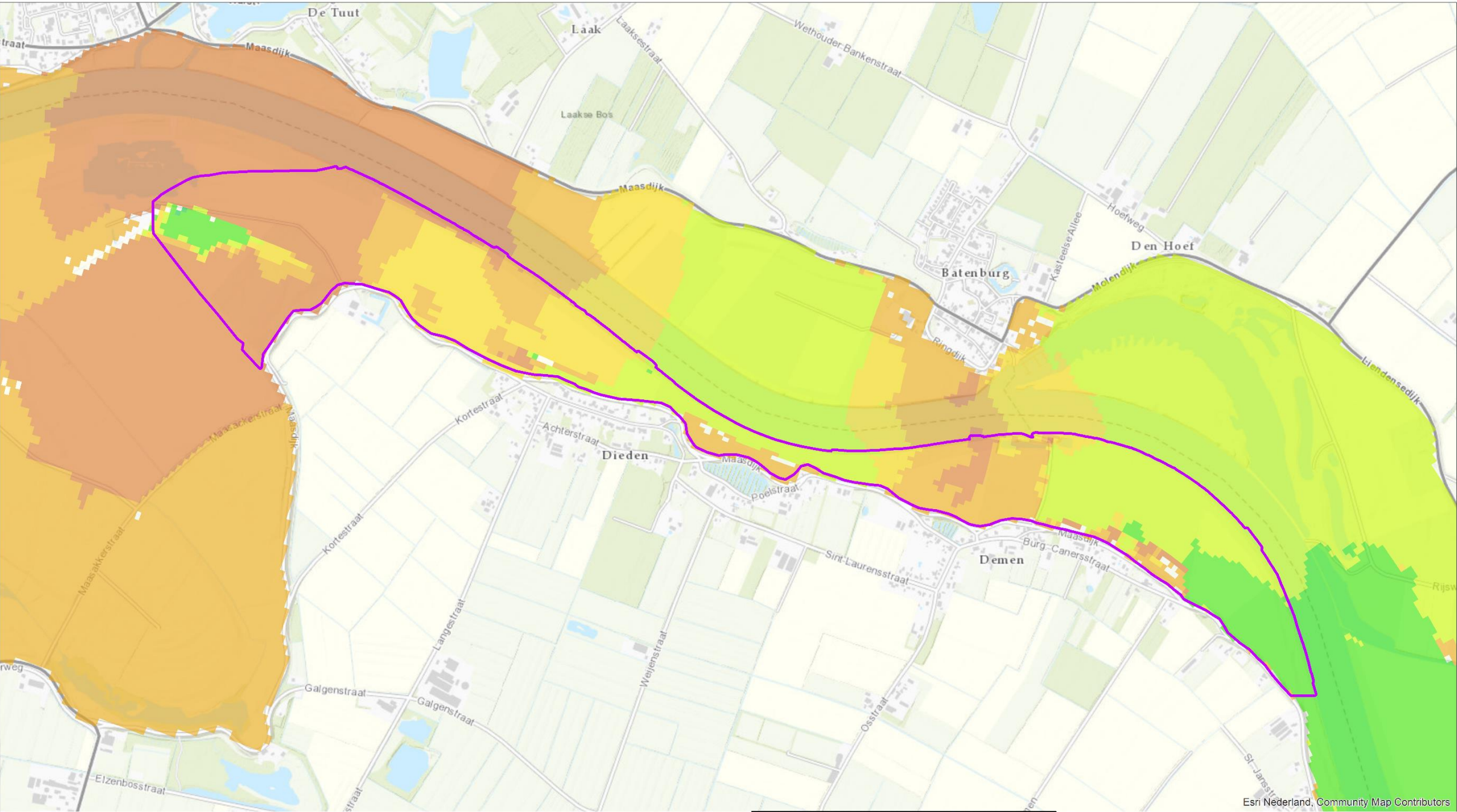
Waterstandverschillen [m] bij 2.000 m³/s
