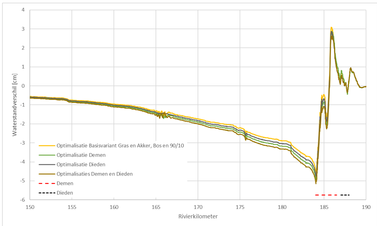
Figuur 11: Derde optimalisatieslag
