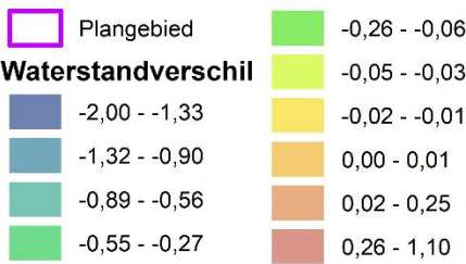
Waterstandverschillen [m] bij 1.500 m³/s
