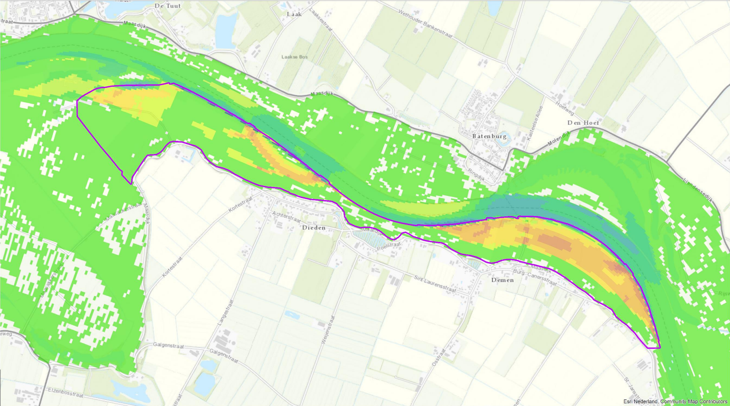
Stroomsnelheidsverschil [m/s] bij 1.250 m³/s
