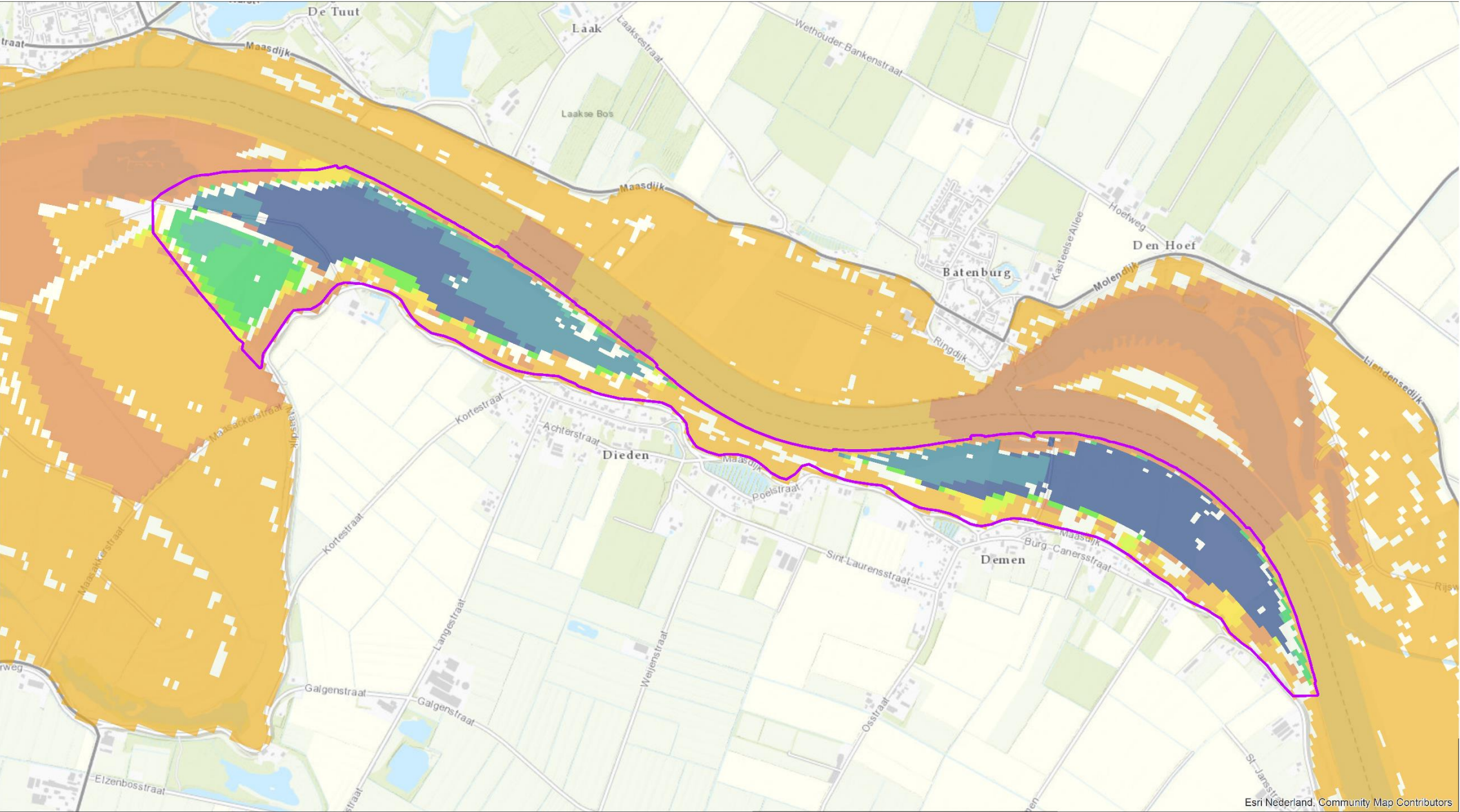
Waterstandverschillen [m] bij 1.250 m³/s
