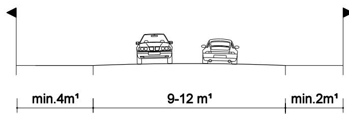
Profiel 3 - schaal 1:200
