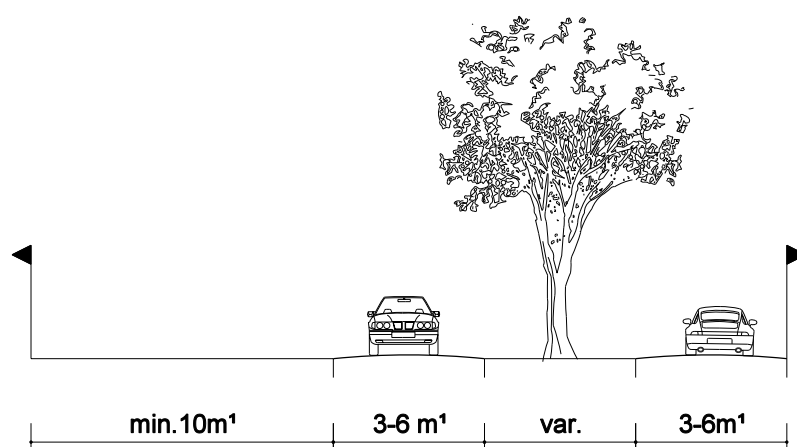
Profiel 1 - schaal 1:200
