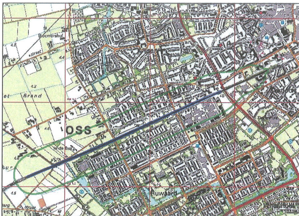
Figuur 4.1: Plaatsgebondenrisicocontouren op basis van de prognosecijfers 2007 met van binnen naar buiten de 10^{-7} /jaar (blauw) en 10^{-8} /jaar (groen) plaatsgebondenrisicocontour
