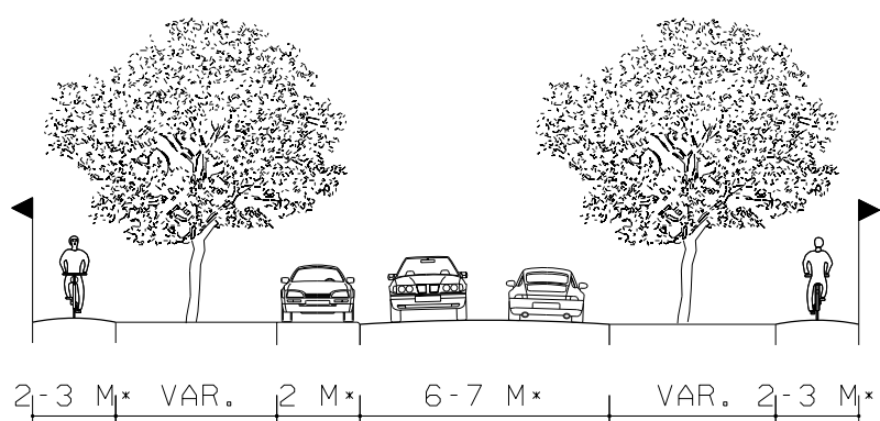
Profiel 4 - schaal 1:200
