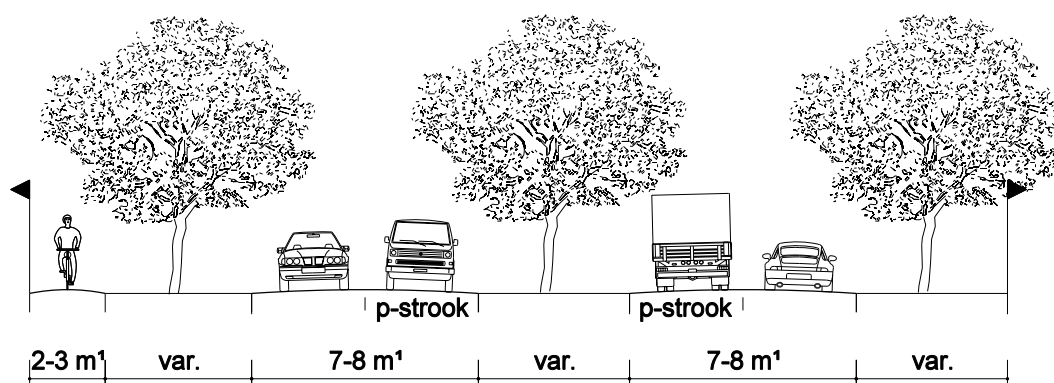
Profiel 4 - schaal 1:200
