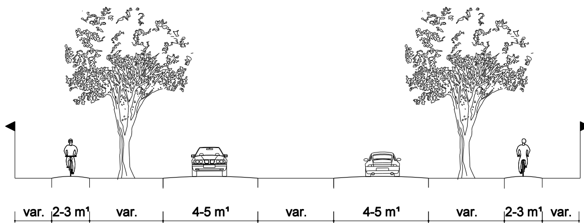
Profiel 3 - schaal 1:200
