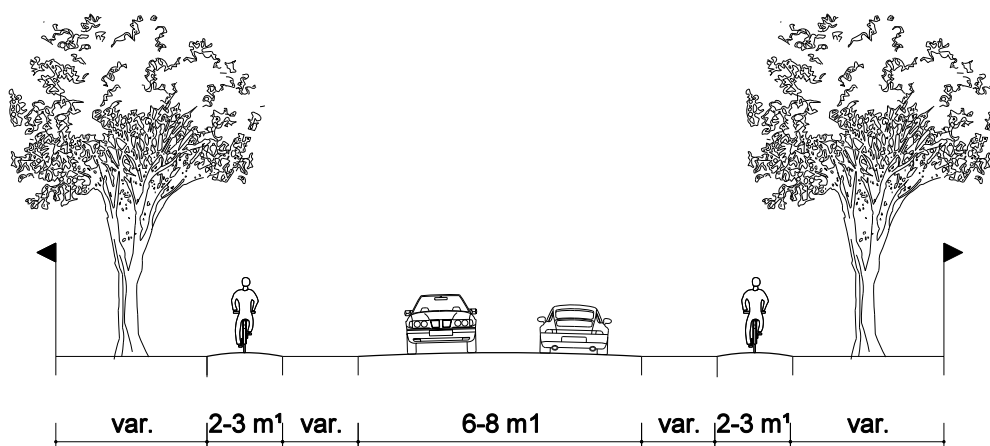
Profiel 2 - schaal 1:200
