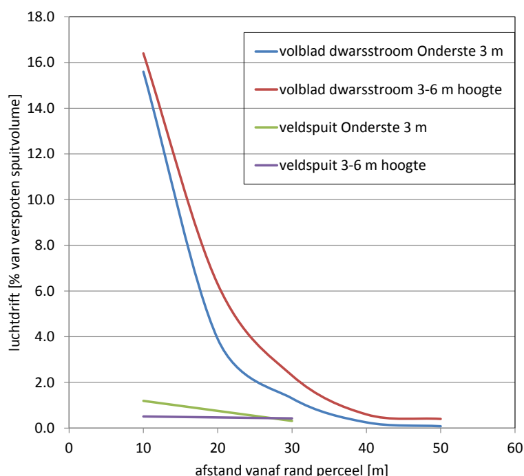
Figuur 7. Vergelijking van de drift naar de lucht (% van de dosering) van standaard fruitteeltspuiten (volblad dwarsstroom) en een veldspuit uitgerust met 50% driftarme spuitdoppen in de lagen 0-3 m en 3-6 m boven grondoppervlak voor verschillende afstanden vanaf de perceelsgrens
