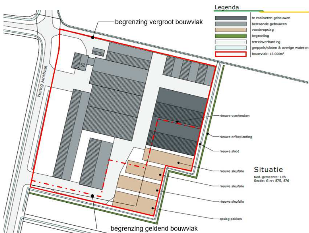
• Figuur 4: Voorlopig ontwerp beoogde situatie (bron: Exlan Advies)
