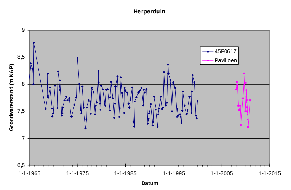
Figuur 17 Grondwaterstandverloop ter plaatse van vakantiepark Herperduin (DINOloket).
