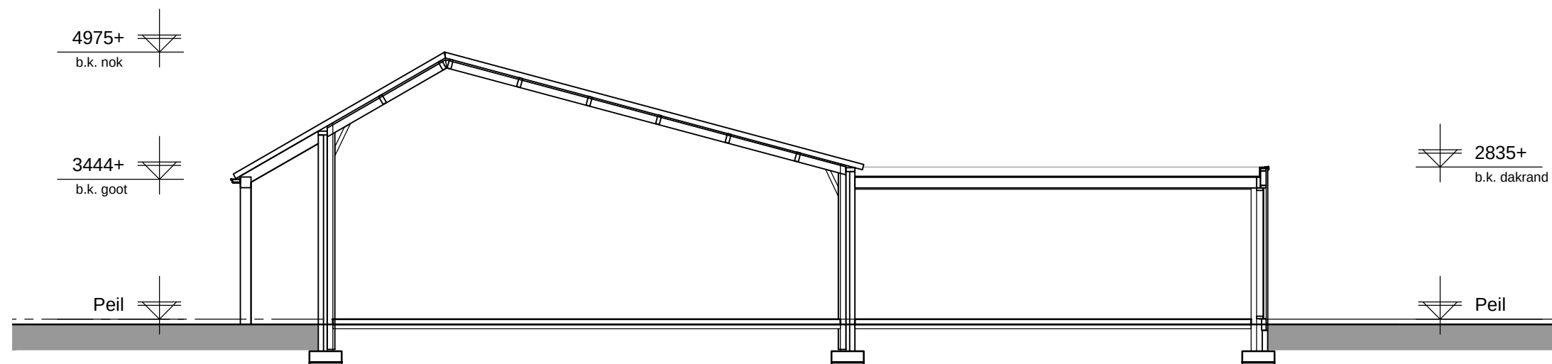
Doorsnede A-A (nieuw)
