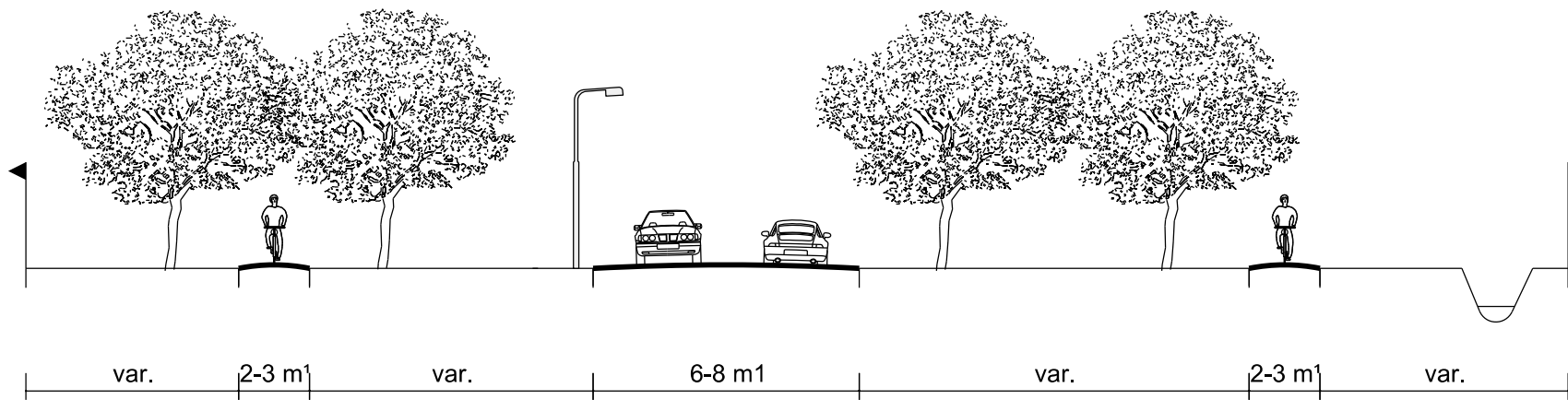
Profiel 15 - St. Sebastianusstraat
