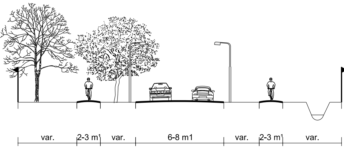
Profiel 11 - Nieuwe Hescheweg
