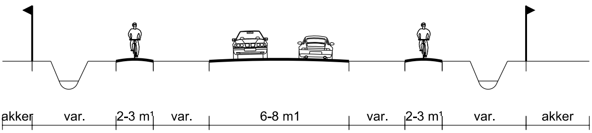
Profiel 5 - John F. Kennedybaan
