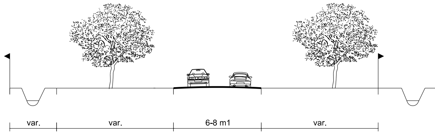
Profiel 16 - Dorpenweg (Overlangel)
