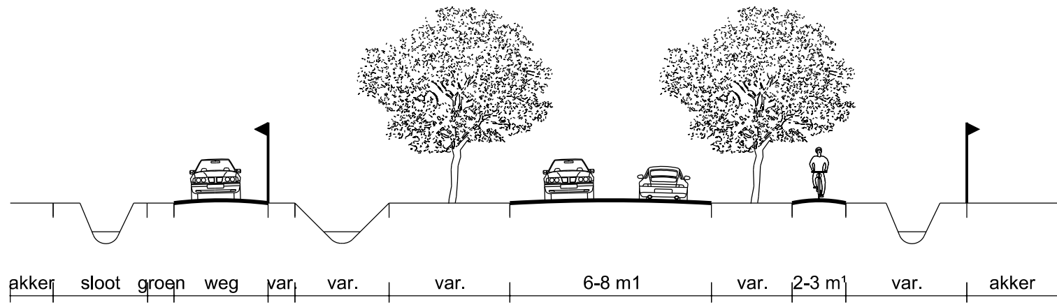
Profiel 7 - Beatrixweg / Hoogveldsestraat
