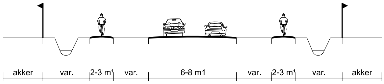
Profiel 9 - Dorpenweg (Deursen-Dennenburg)
