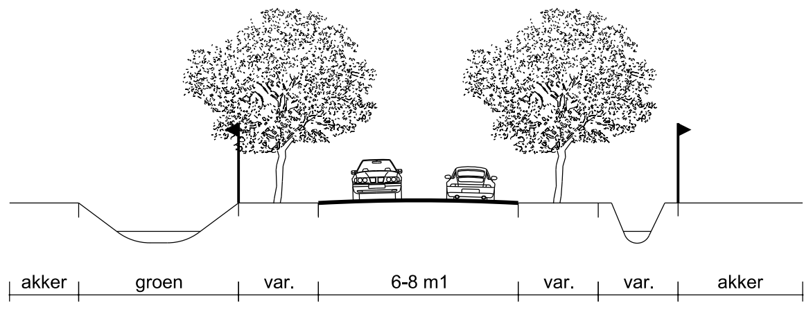
Profiel 3 - Mr. van Coothstraat
