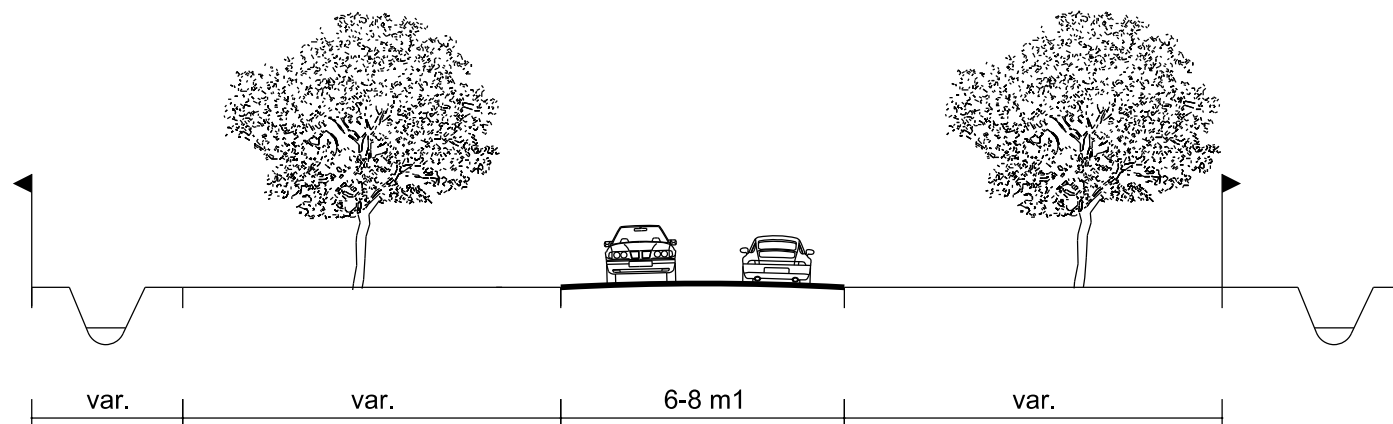
Profiel 16 - schaal 1:200
