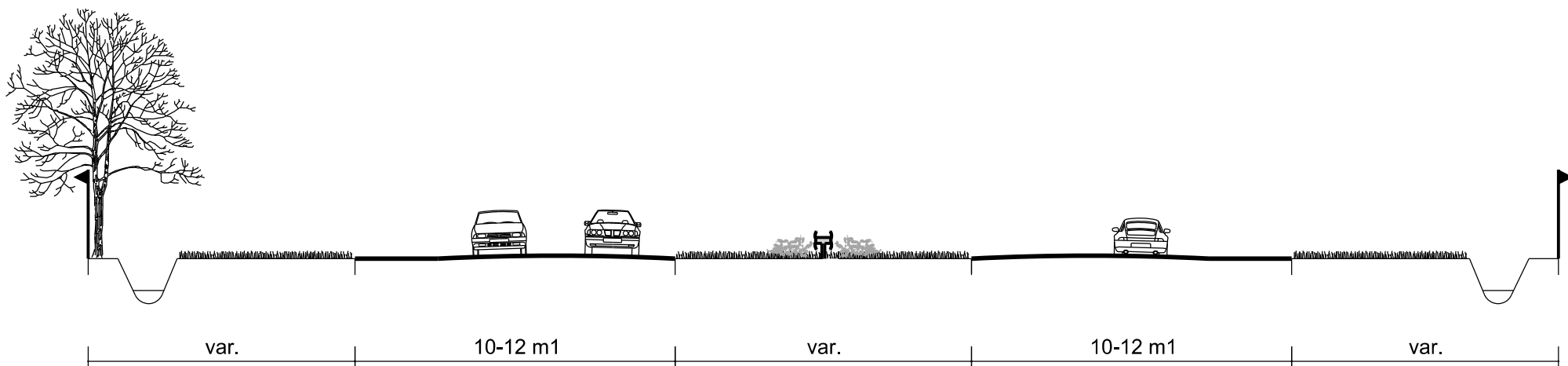
Profiel 14 - schaal 1:200
