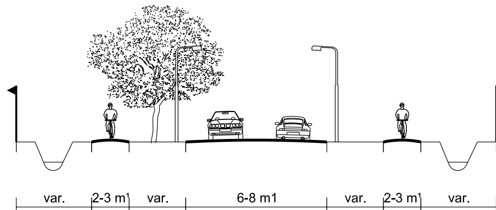
Profiel 13 - schaal 1:200
