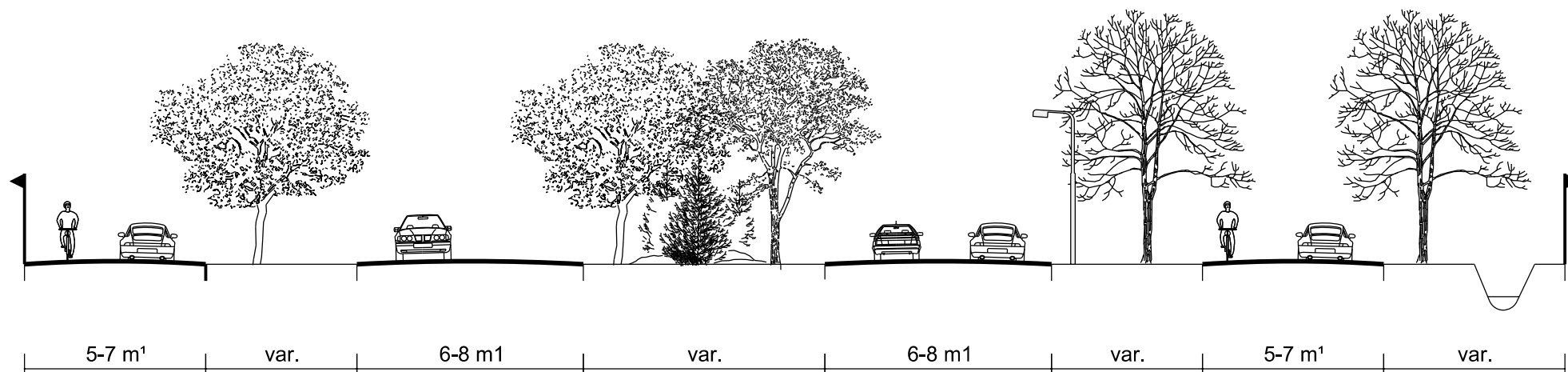
Profiel 10 - schaal 1:200
