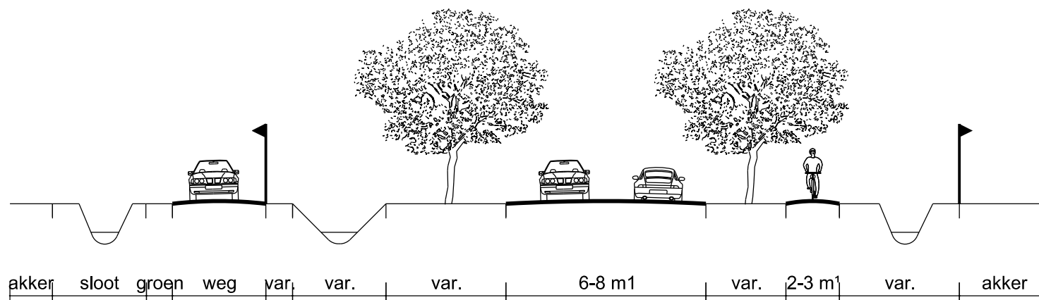
Profiel 7 - schaal 1:200
