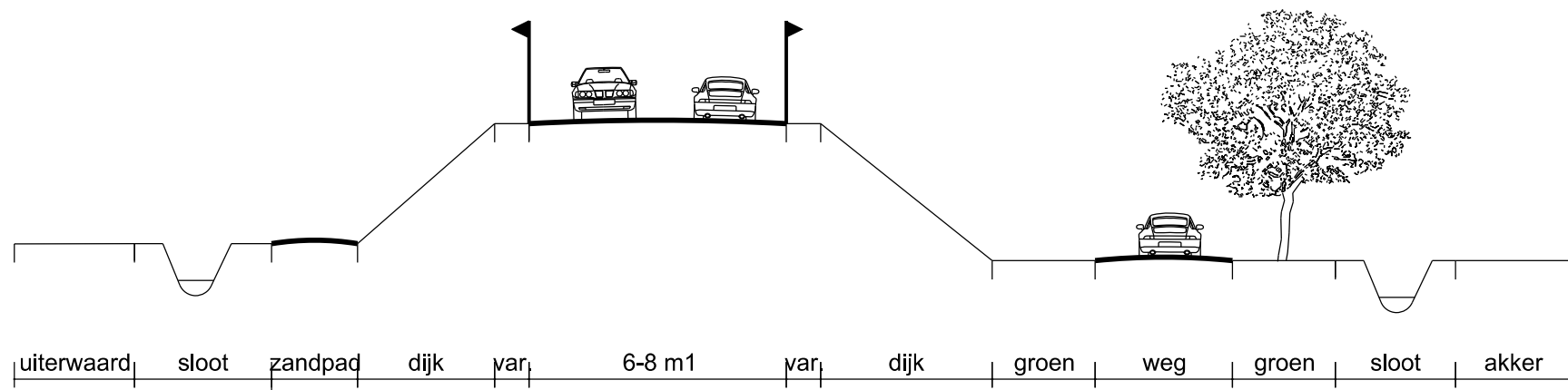
Profiel 2 - schaal 1:200
