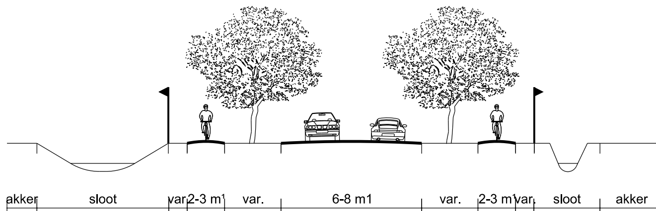
Profiel 1 - schaal 1:200
