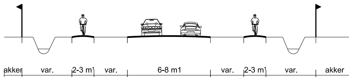
Profiel 5 - schaal 1:200
