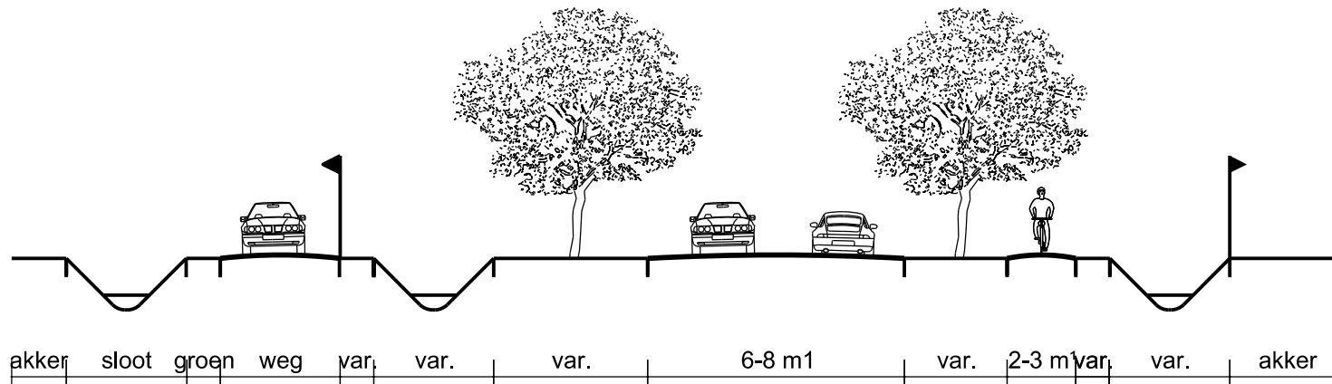
Profiel 7 - schaal 1:200
