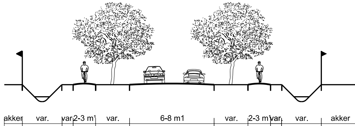
Profiel 6 - schaal 1:200
