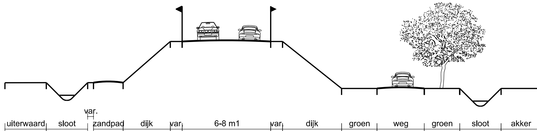
Profiel 2 - schaal 1:200
