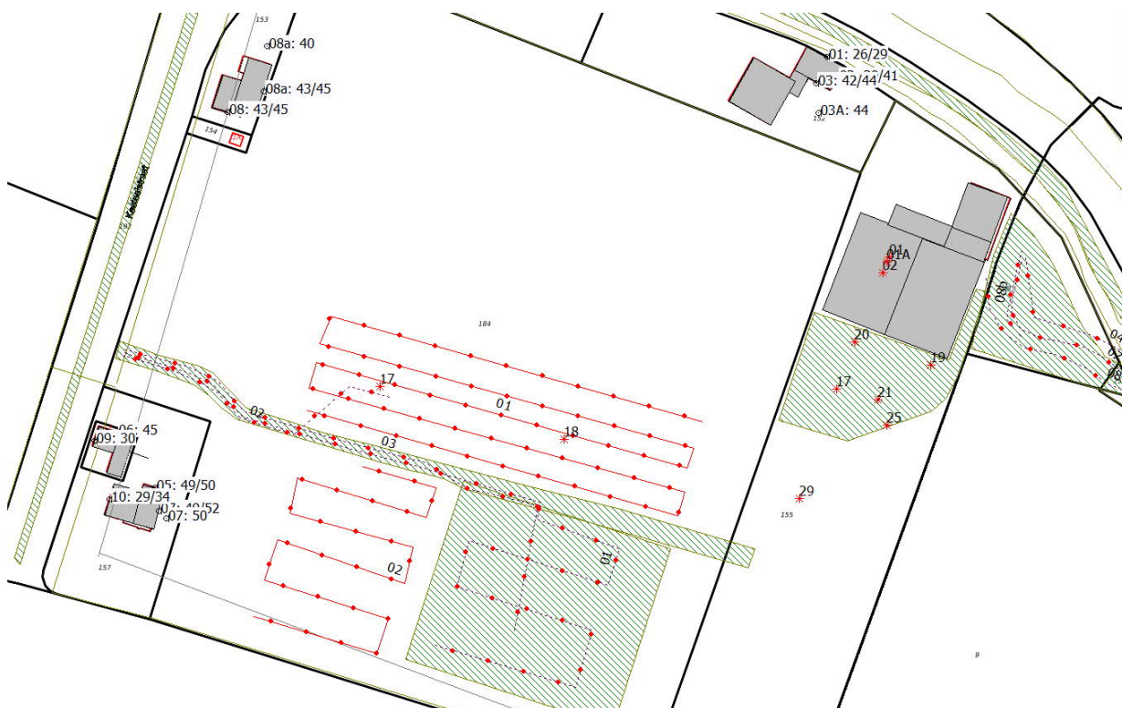
Figuur 3: Directe hinder L_{ArLT} , dagperiode RBS 2 maaien
