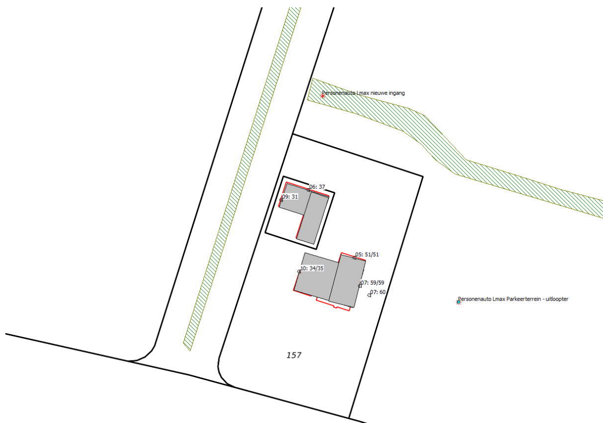
Figuur 7: Directe hinder L_{Amax} , nachtperiode rondom Kasteelstraat 4 t.g.v. autoportier (bron 31).
