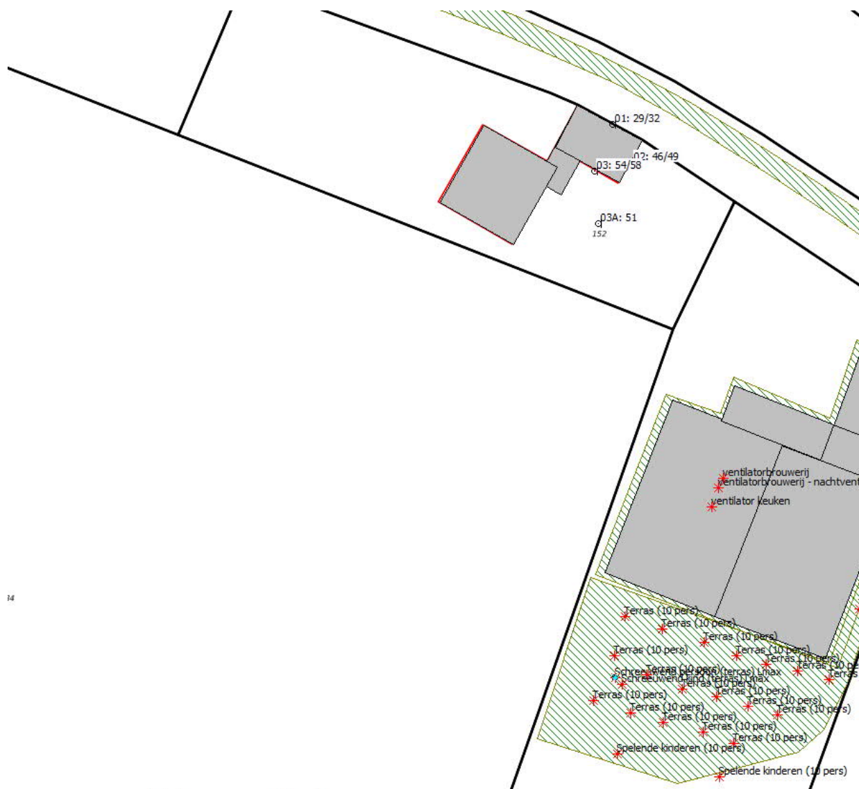
Figuur 5: Directe hinder L_{Amax} , nachtperiode rondom Oijense Bovendijk 59 t.g.v. schreeuwende terrasbezoeker (bron 31).
