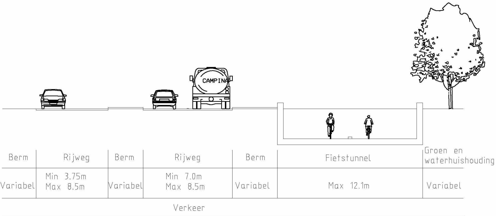
Dwarsprofiel B-B
