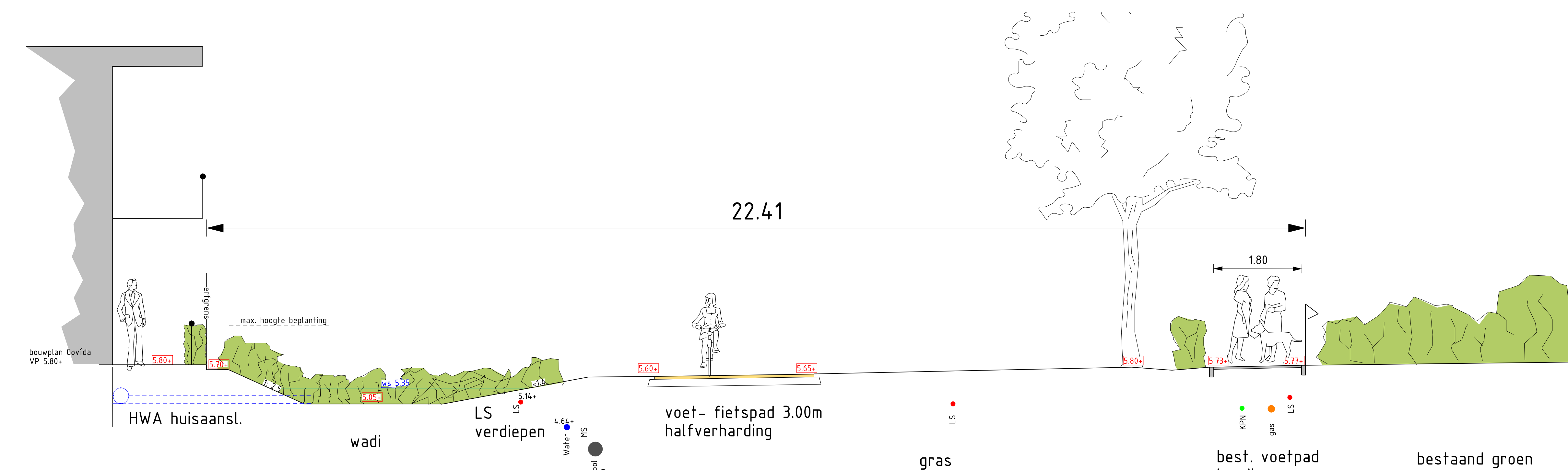
DOORSNEDE A-A 1 : 50
