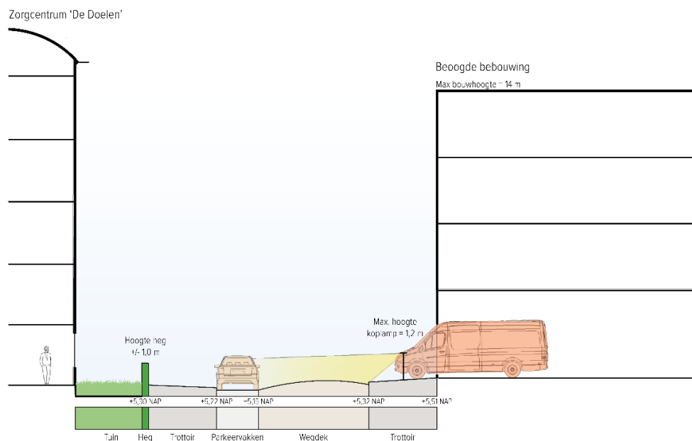
Figuur 4: Lichthinder bij maximale koplamphoogte
