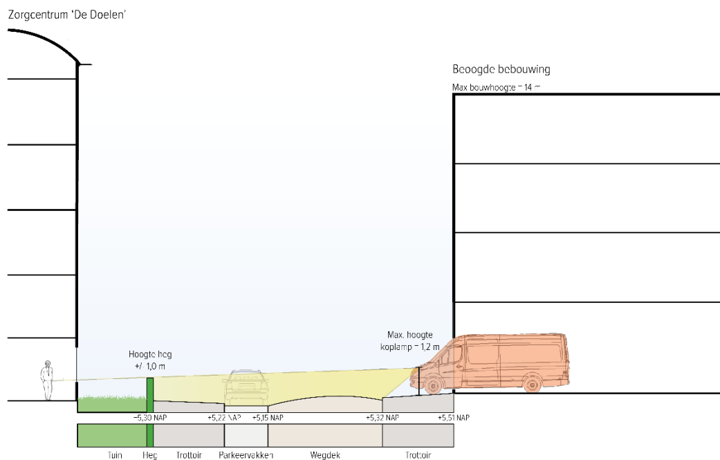
Figuur 5: Lichthinder bij maximale koplamphoogte
