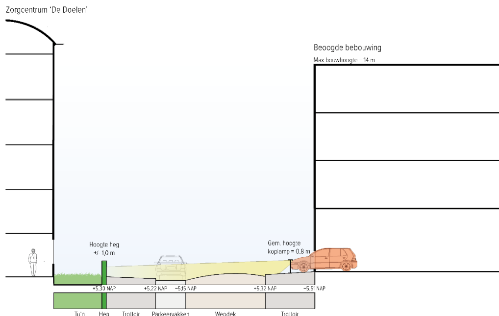
Figuur 2: Lichthinder bij een gemiddelde koplamphoogte
