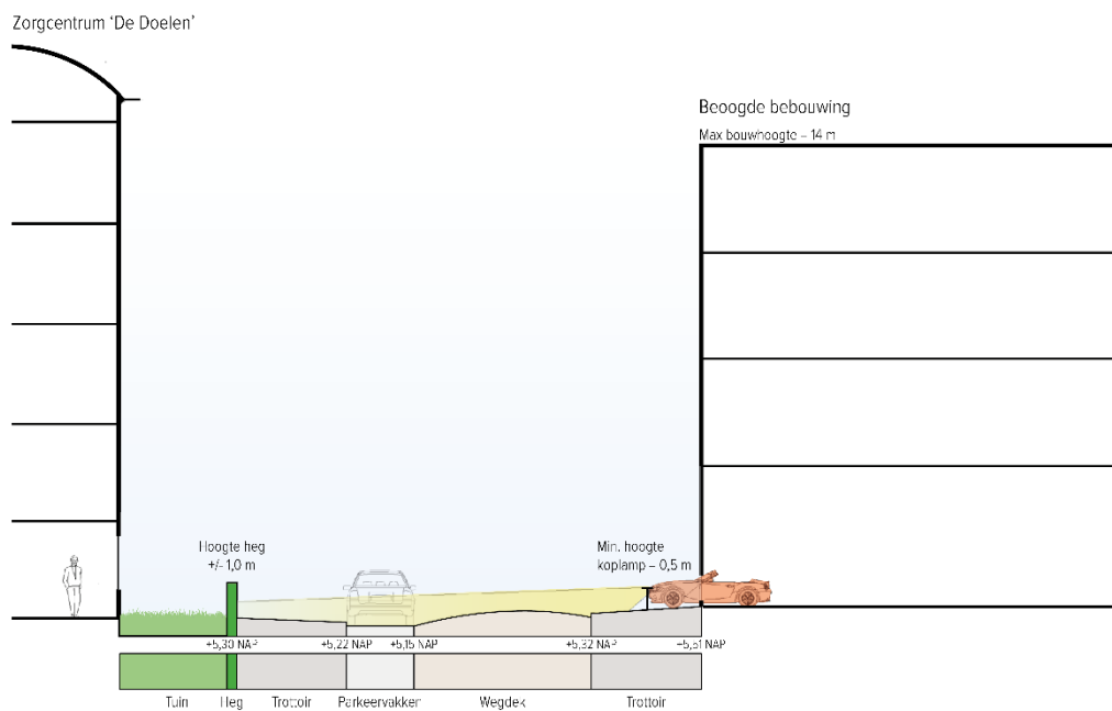
Figuur 3: Lichthinder bij de minimale koplamphoogte
