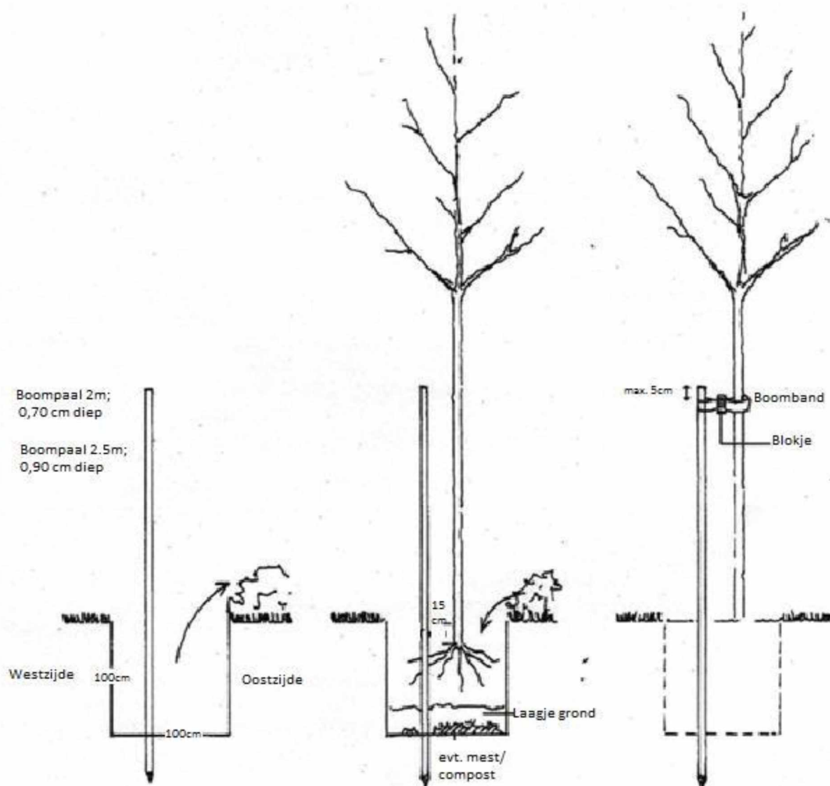
Afbeelding 5: Plantinstructie bomen
