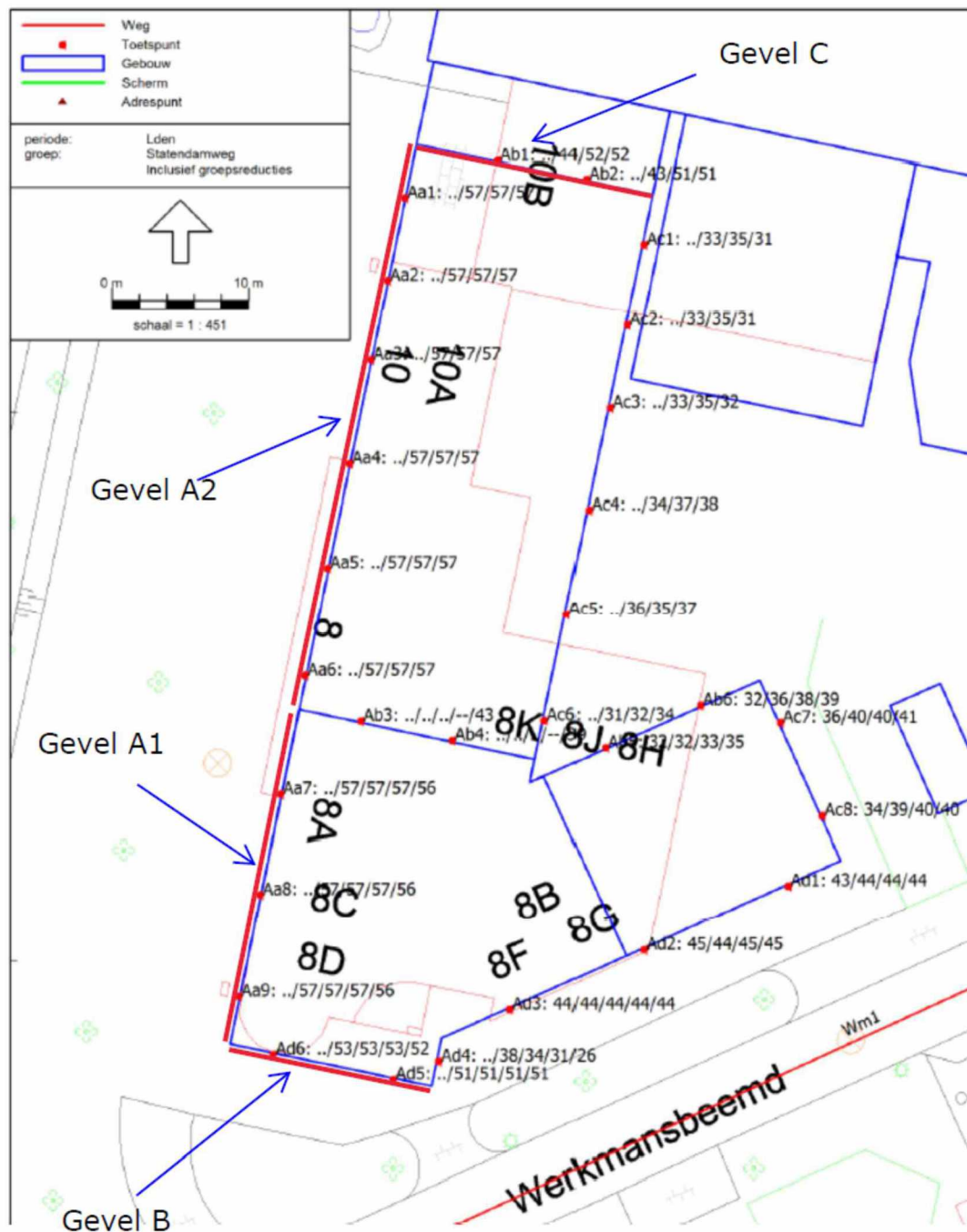
Figuur 2 Gevel A1, A2, B en C (verkeerslawaai Statendamweg, zonder maatregel, incl. aftrekcorrectie)
