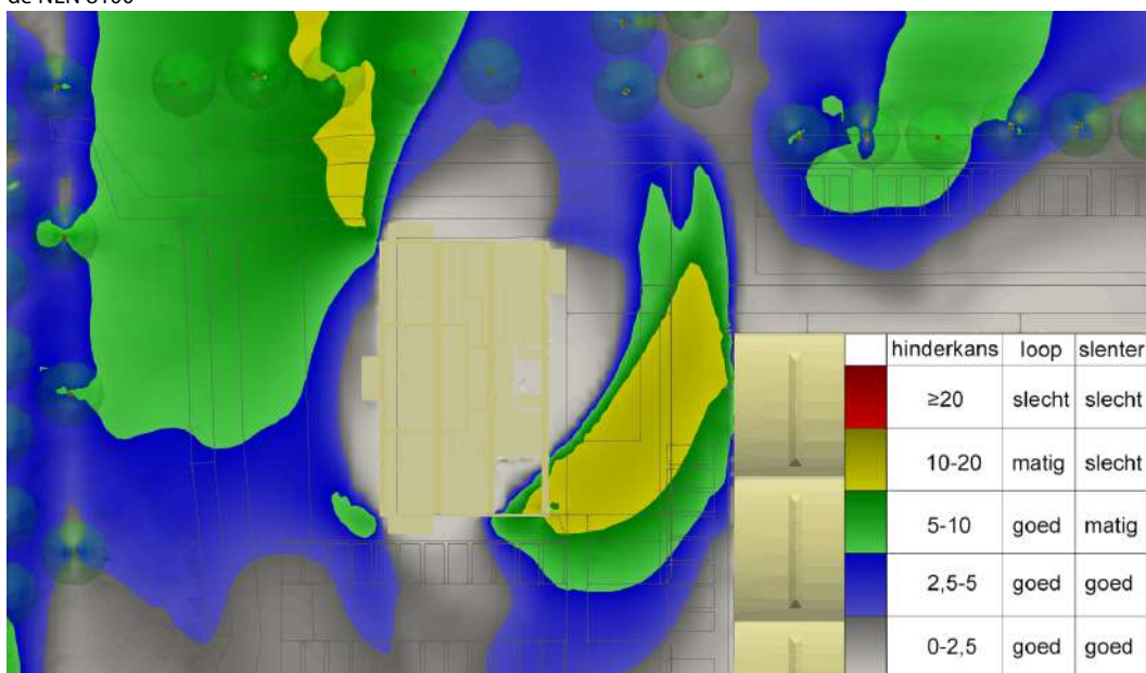
f3.3 Het te verwachten windklimaat rond de westelijke toren in de geplande bebouwingssituatie, beoordeeld volgens de NEN 8100
