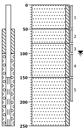
Boring: 901 Datum: 15-03-2016
