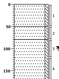
Boring: 904 Datum: 15-03-2016
