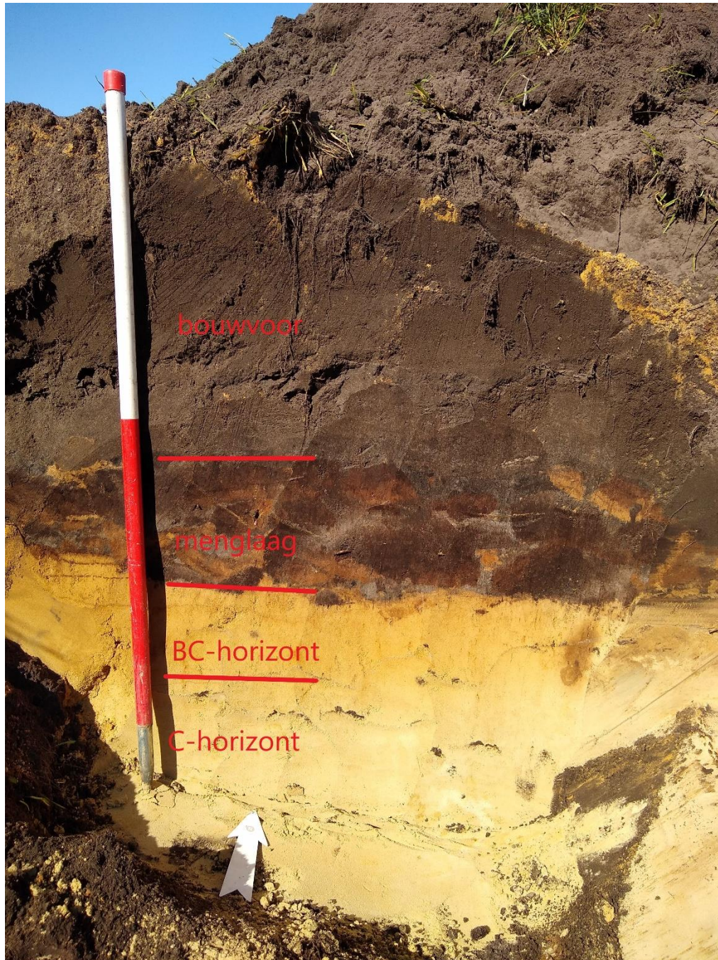
Figuur 5. Representatief profiel (profiel 1212) met een bouwvoor, menglaag/gebroken podzol, BC-horizont en C-horizont.
