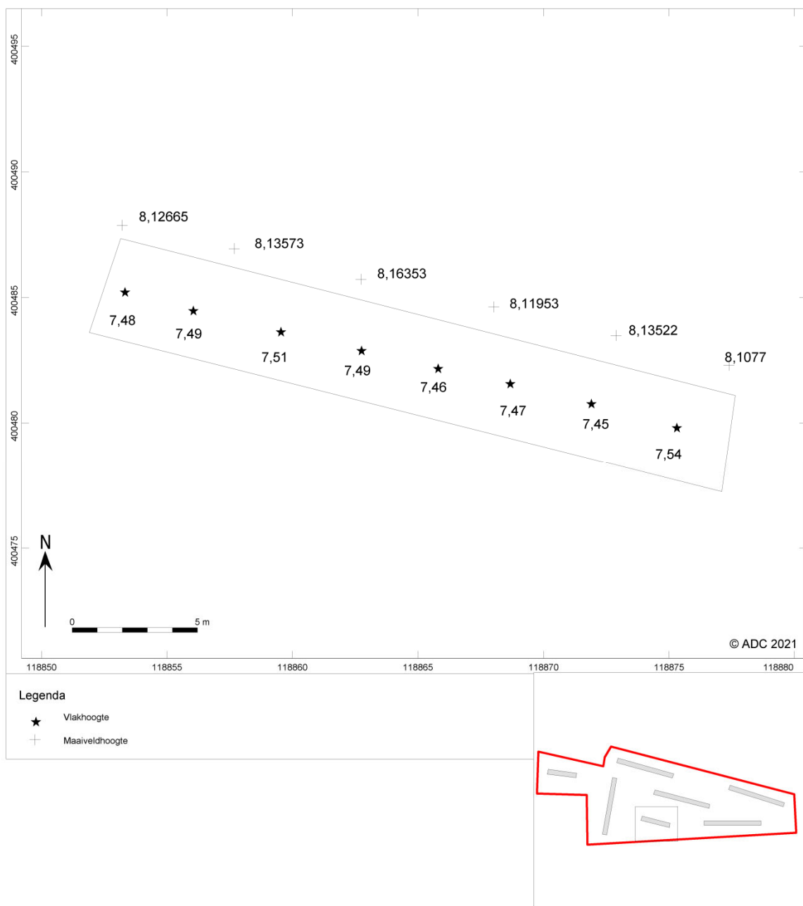
Sleuf 4
