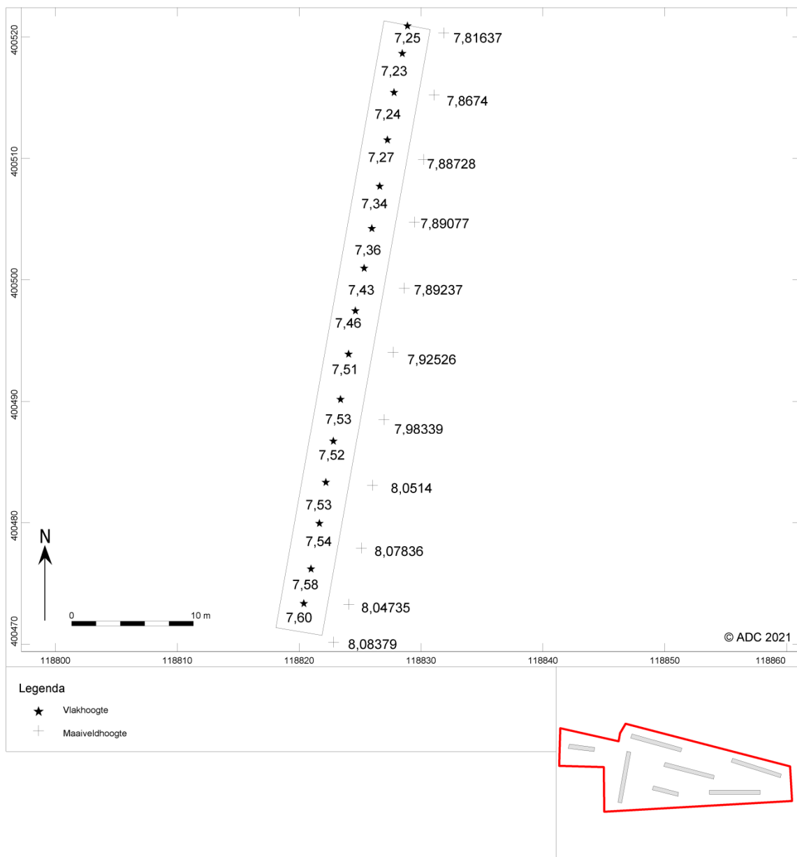
Sleuf 3
