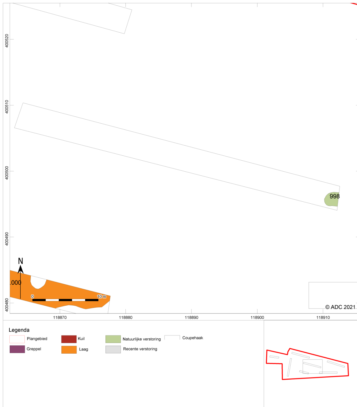
Sleuf 5
