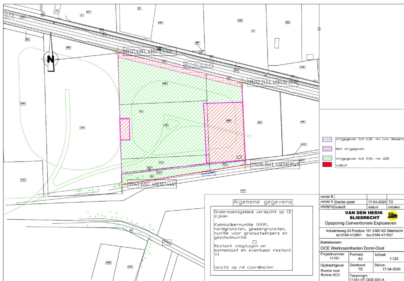
Figuur 4 – vrijgavetekening
