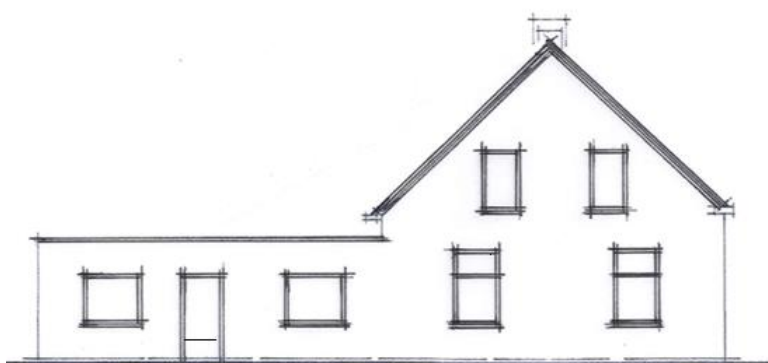
ZIJGEVEL LINKS
