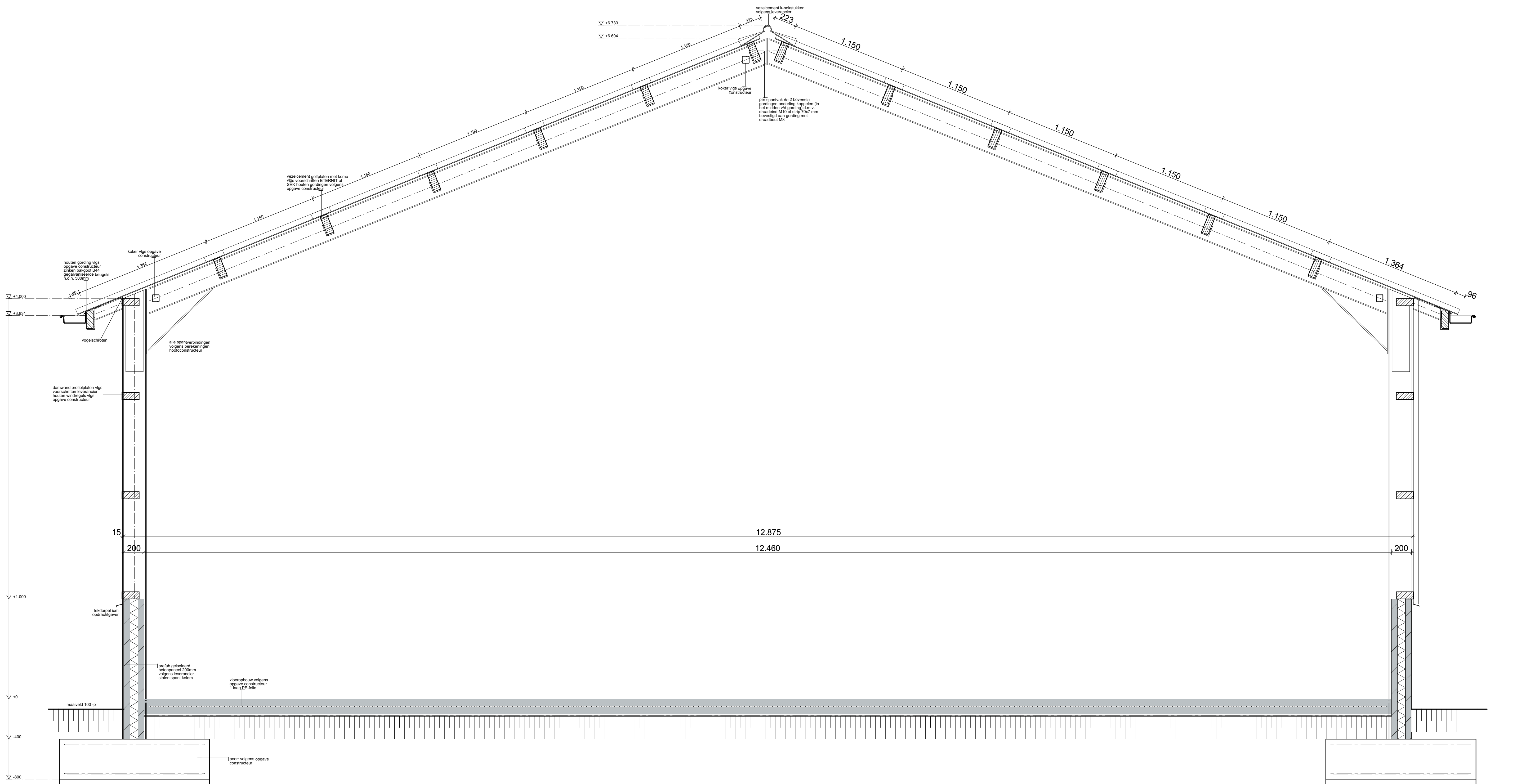
DOORSNEDE A-A
