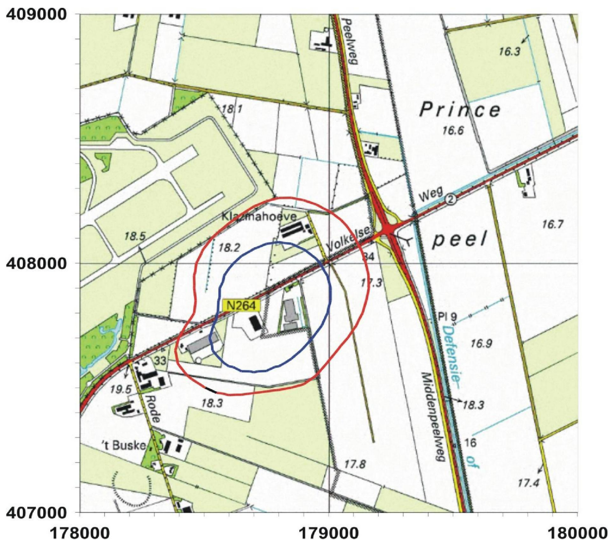
Figuur 5.1. Geurcontouren van 0,5 (rood) en 1 (blauw) \text{ou}_E(\text{H})/\text{m}^3 als 98-percentiel
