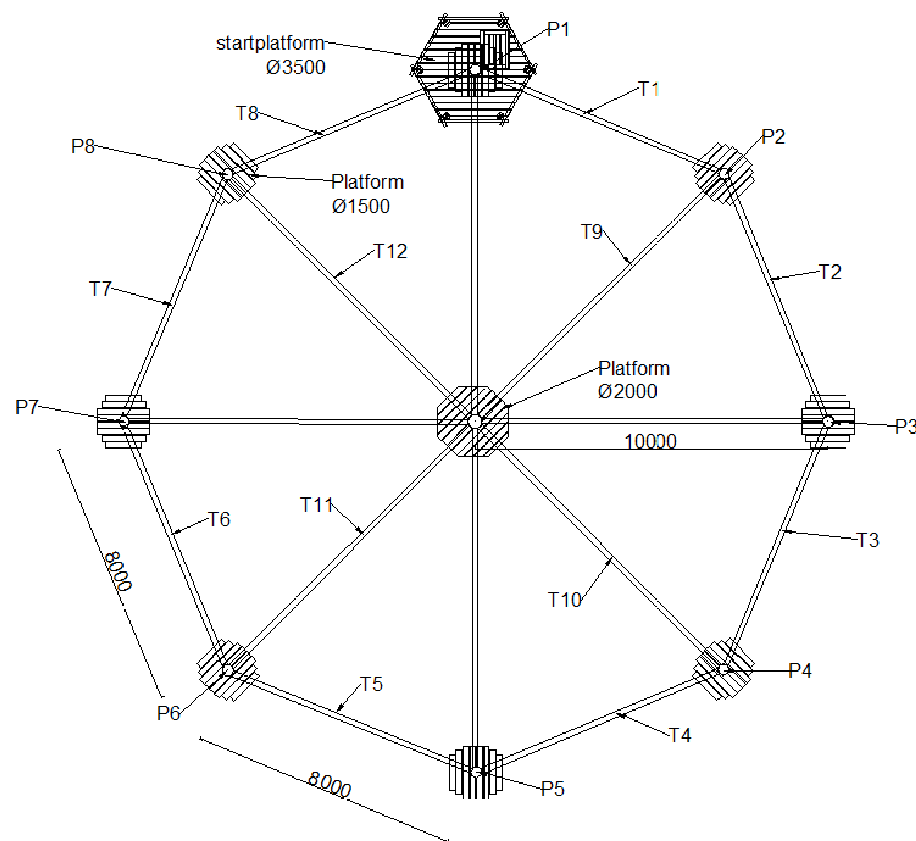
BOVENAANZICHT KLIMPARK
