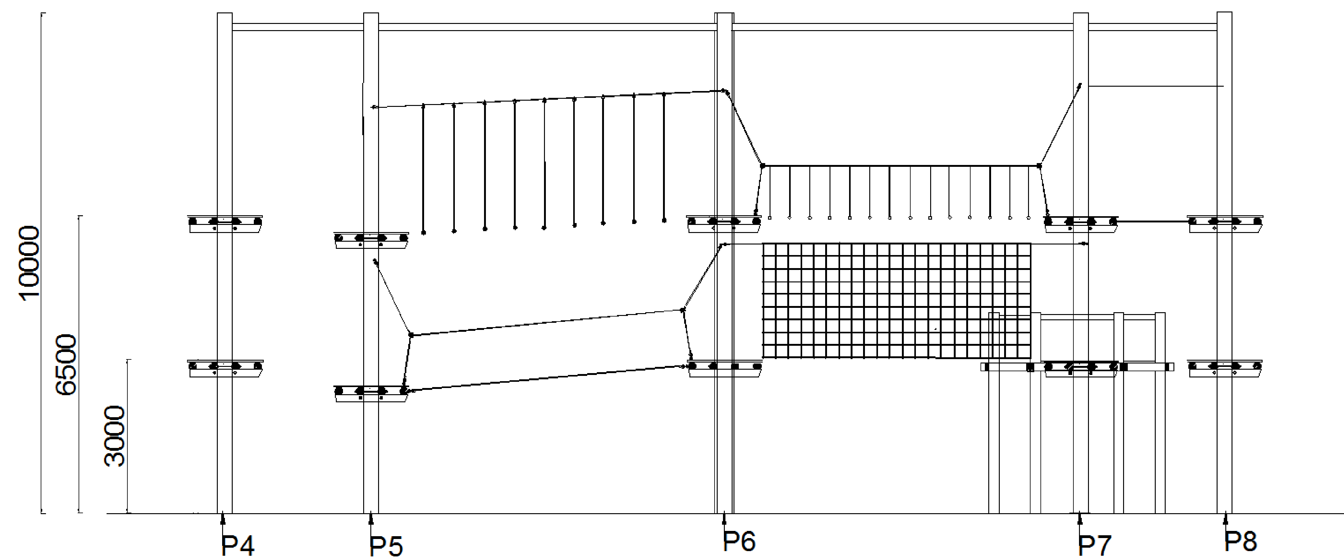
VOORAANZICHT KLIMPARK
