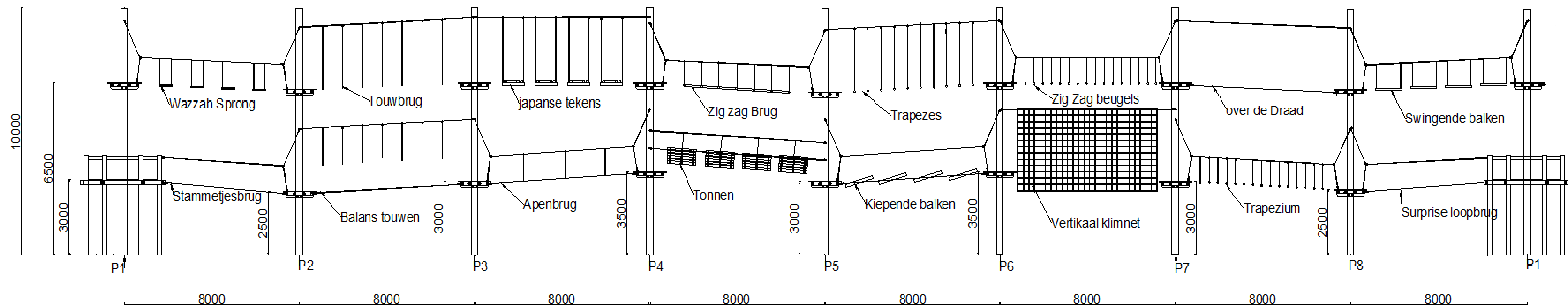
UITGEKLAPTE AANZICHT KLIMPARK
