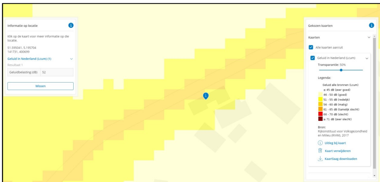
Afbeelding 21: uitsnede geluidbelasting
