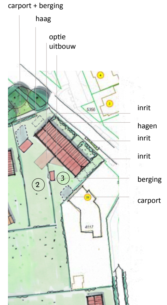
uitsnede stedenbouwkundig plan, kavelgrenzen, plaatsing bijgebouwen indicatief weergegeven
