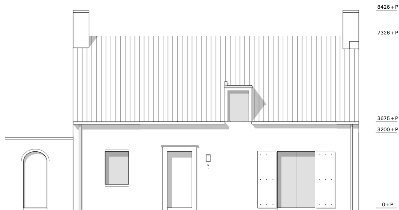
VOORGEVEL
