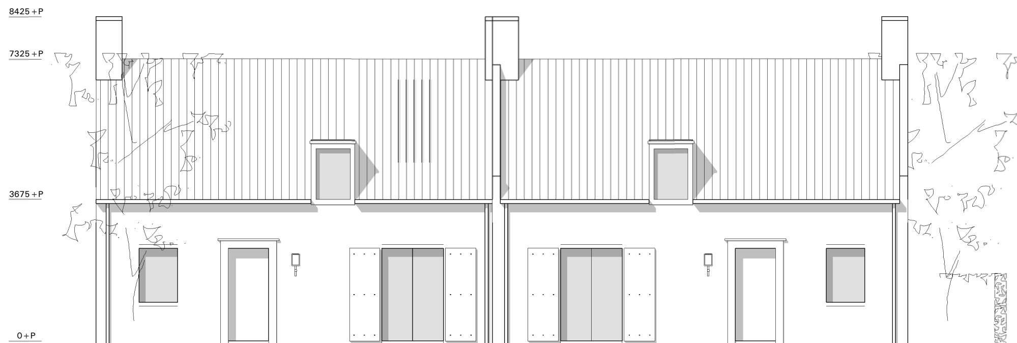
VOORGEVEL
