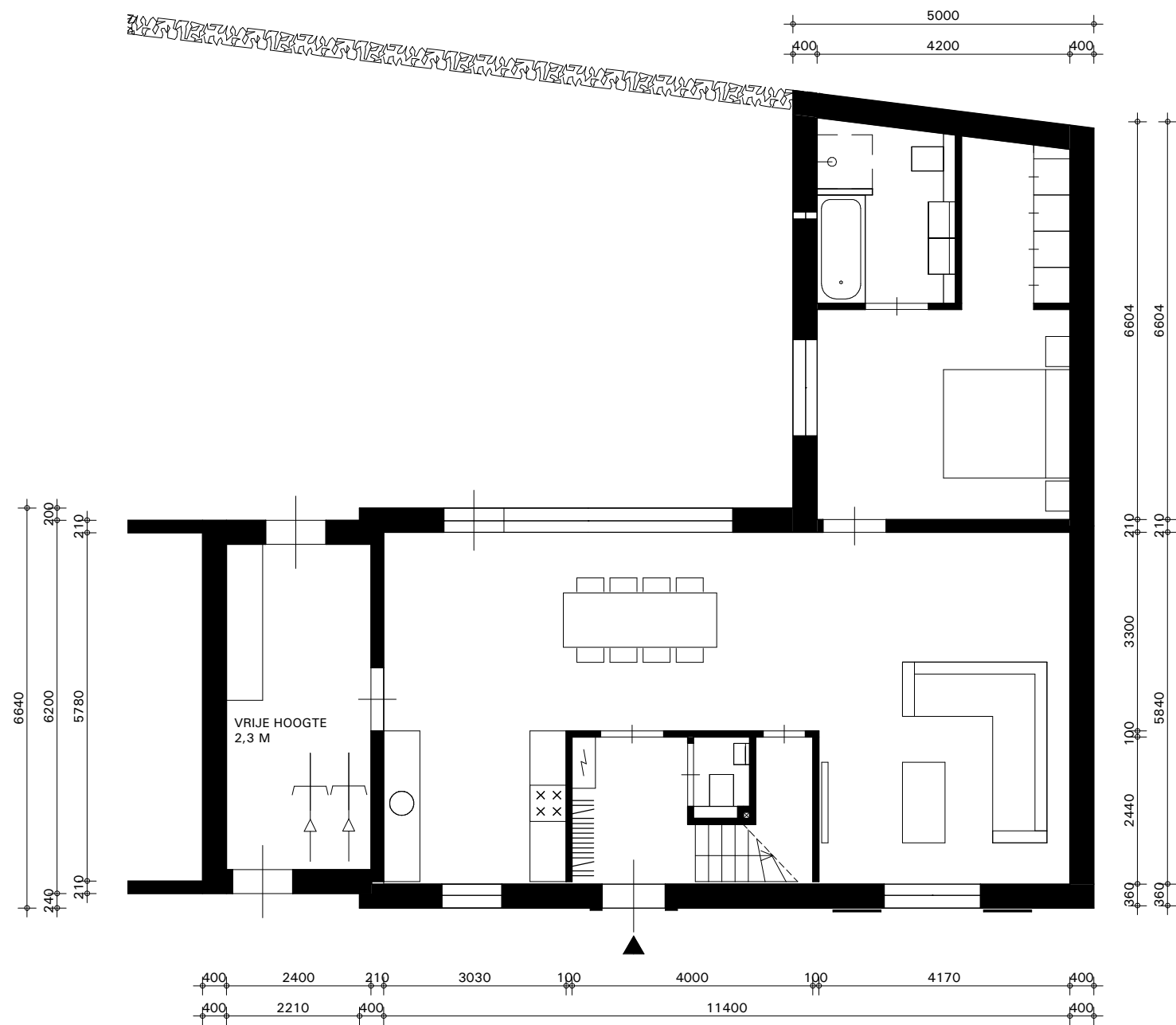
BEGANE GROND
