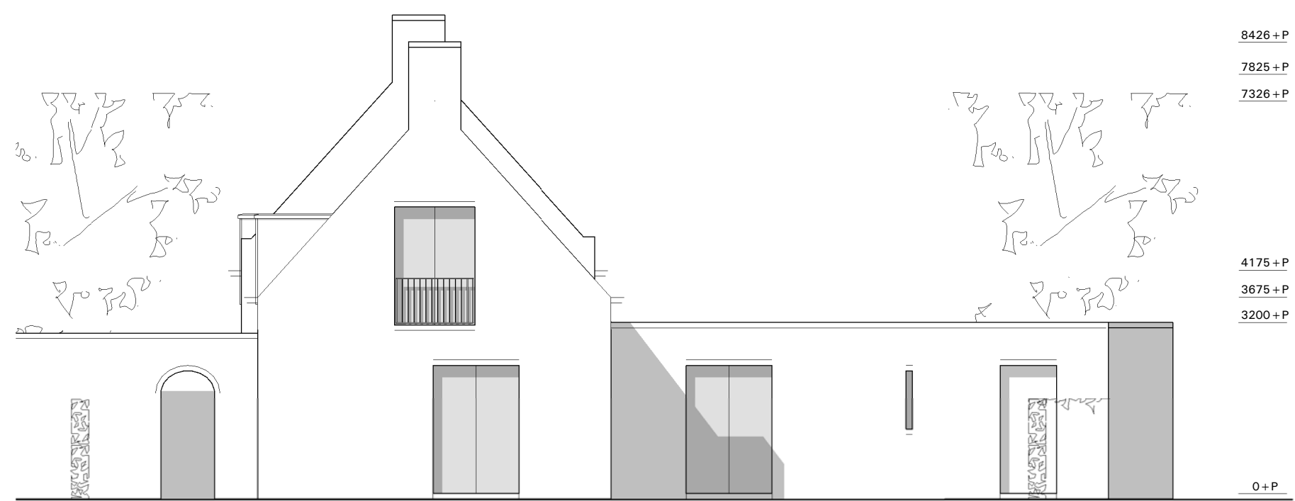
RECHTERGEVEL
