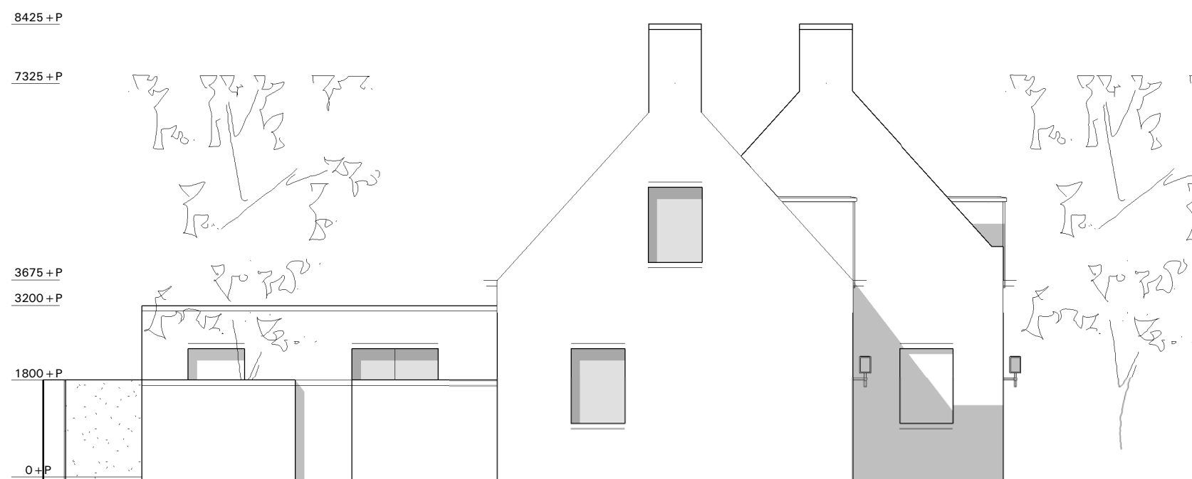
LINKERGEVEL
